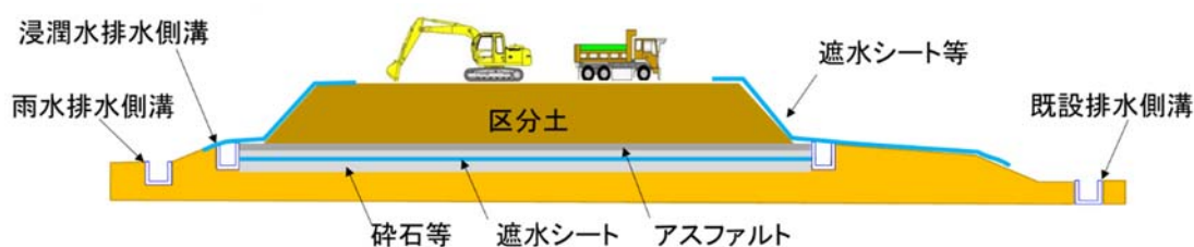
図 5-3 湯島地区（南草里）発生土仮置き場における計画（区分土搬入中）
