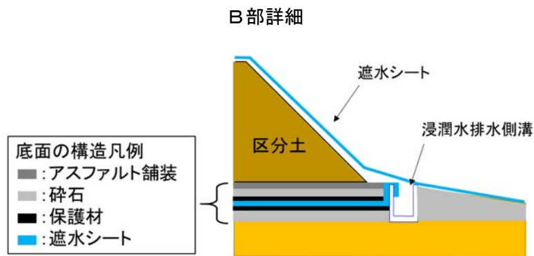
図 2-3(2) 湯島地区（南草里）発生土仮置き場における盛土計画
