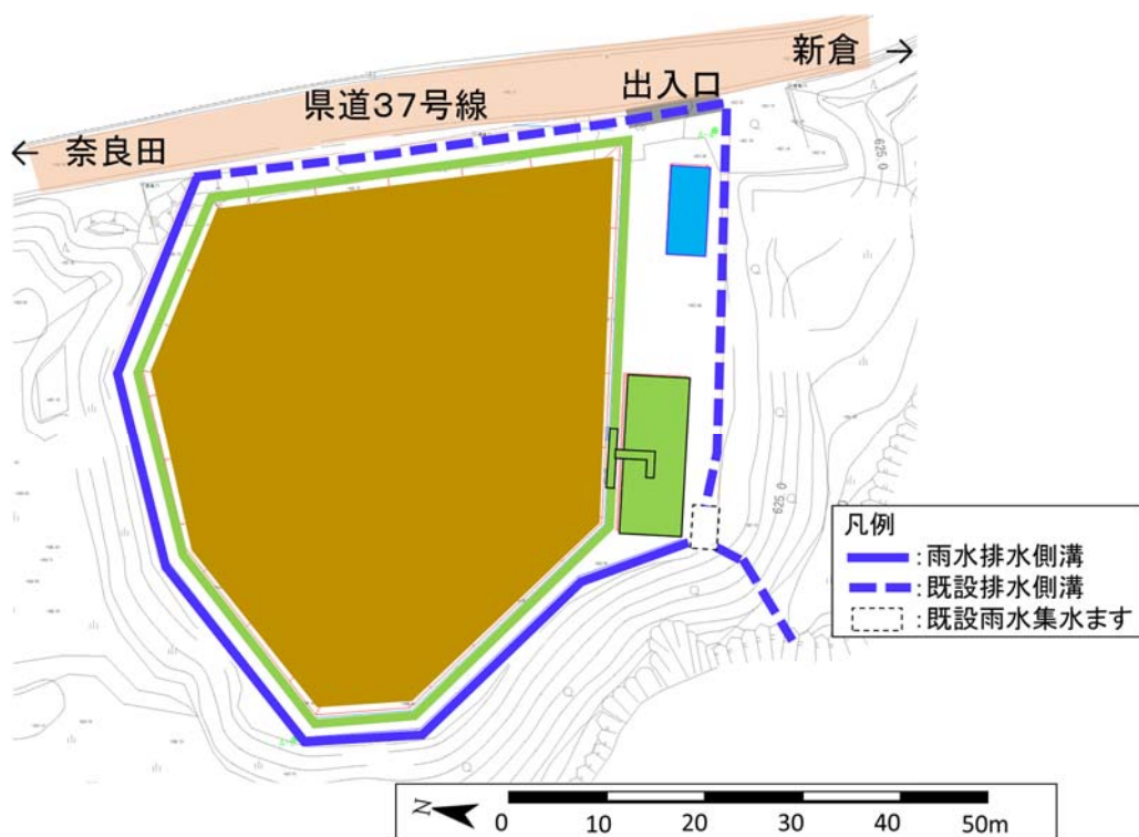
図 5-2 湯島地区（南草里）発生土仮置き場の雨水側溝
