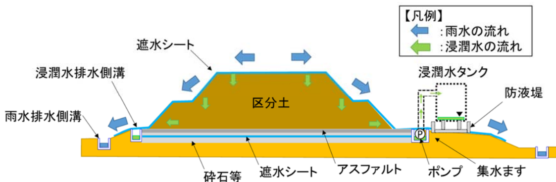
図5-4 湯島地区（南草里）発生土仮置き場における計画（仮置き期間中）
