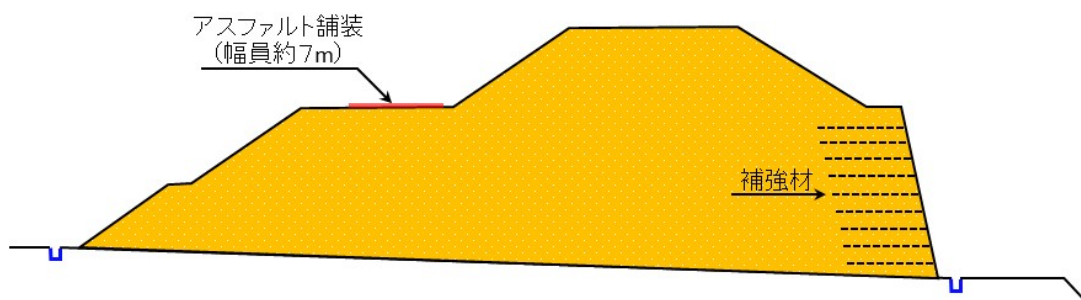
図2-4 (2) 塩島地区（河川側）発生土仮置き場における主な施工手順（仮置き）
