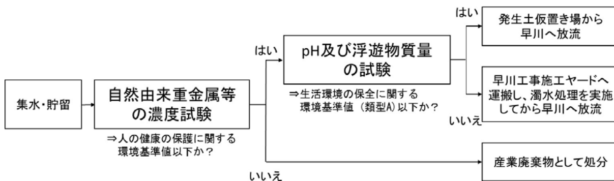
図 4-1-1-2 塩島地区（下流）発生土仮置き場の排水処理フロー
