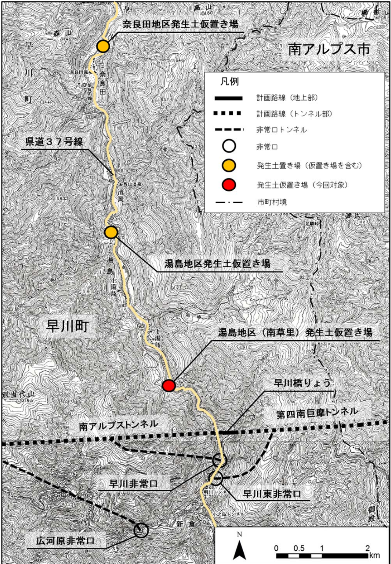
図 1-1-1(1) 工事位置図
