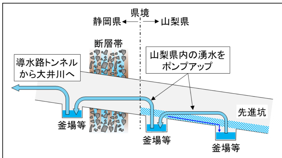
図 1 山梨県内で発生するトンネル湧水を先進坑貫通後に大井川に戻す方策
