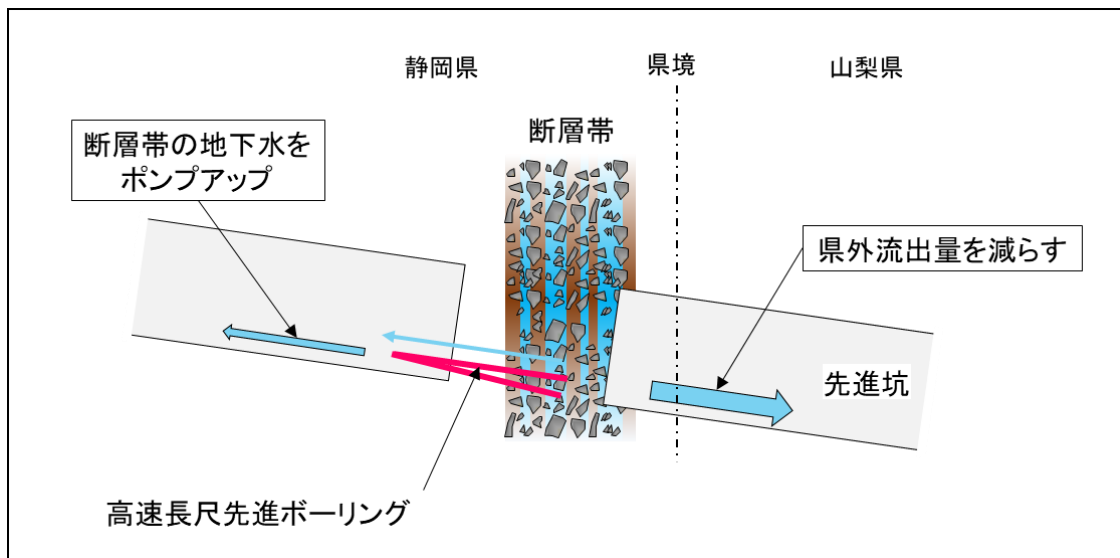
図 4 県外流出量をできる限り減らす方策（山梨県側の例）
