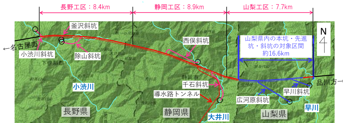
図2 山梨県内で発生するトンネル湧水をポンプアップする区間
