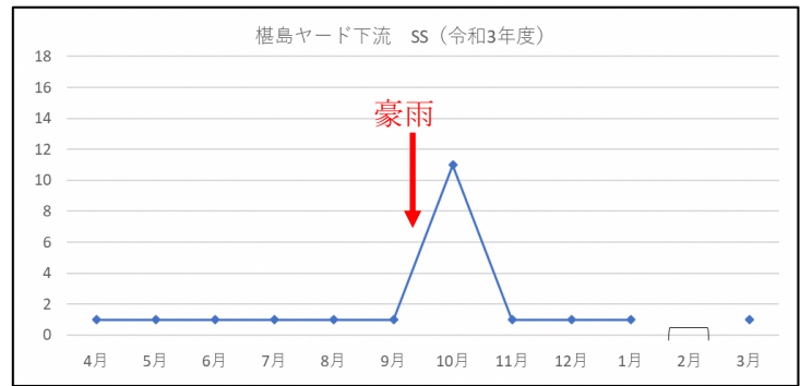
図 1 5 豪雨により濁りが発生した測定例
