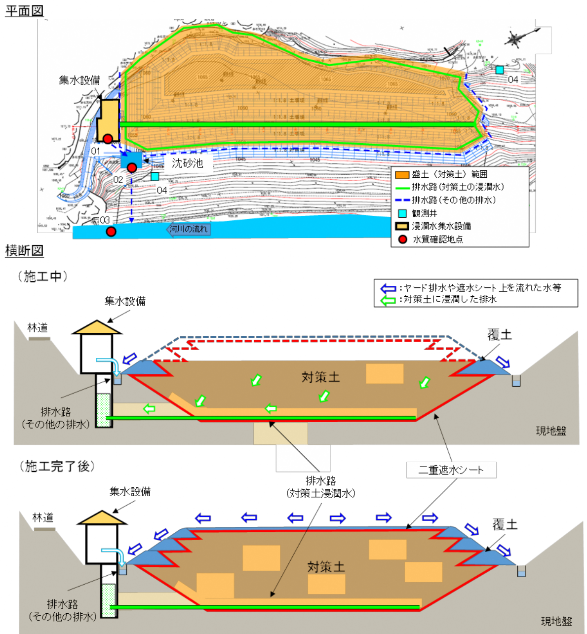
図 7 排水処理計画（イメージ）
