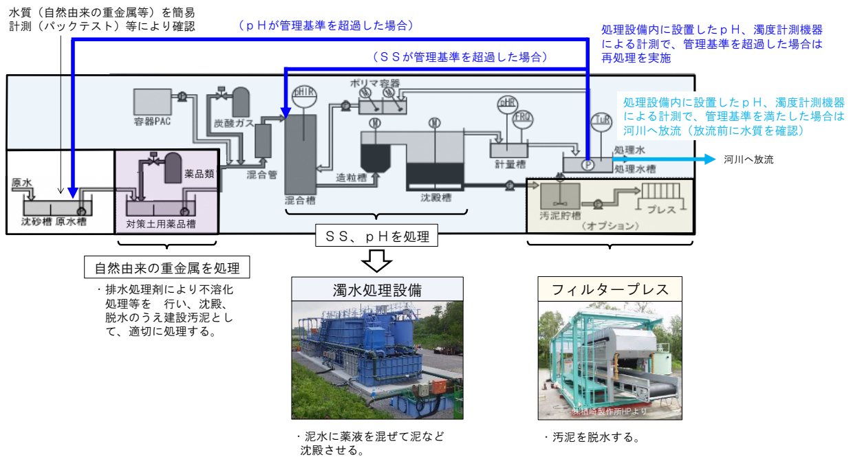
図 18 処理設備による処理のフロー（イメージ）
