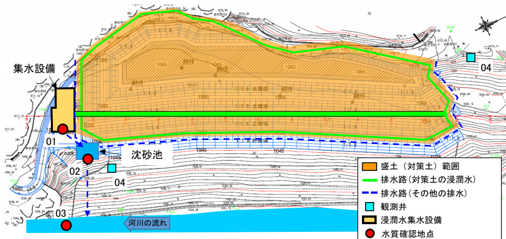
図 22 水質の調査計画（イメージ）
