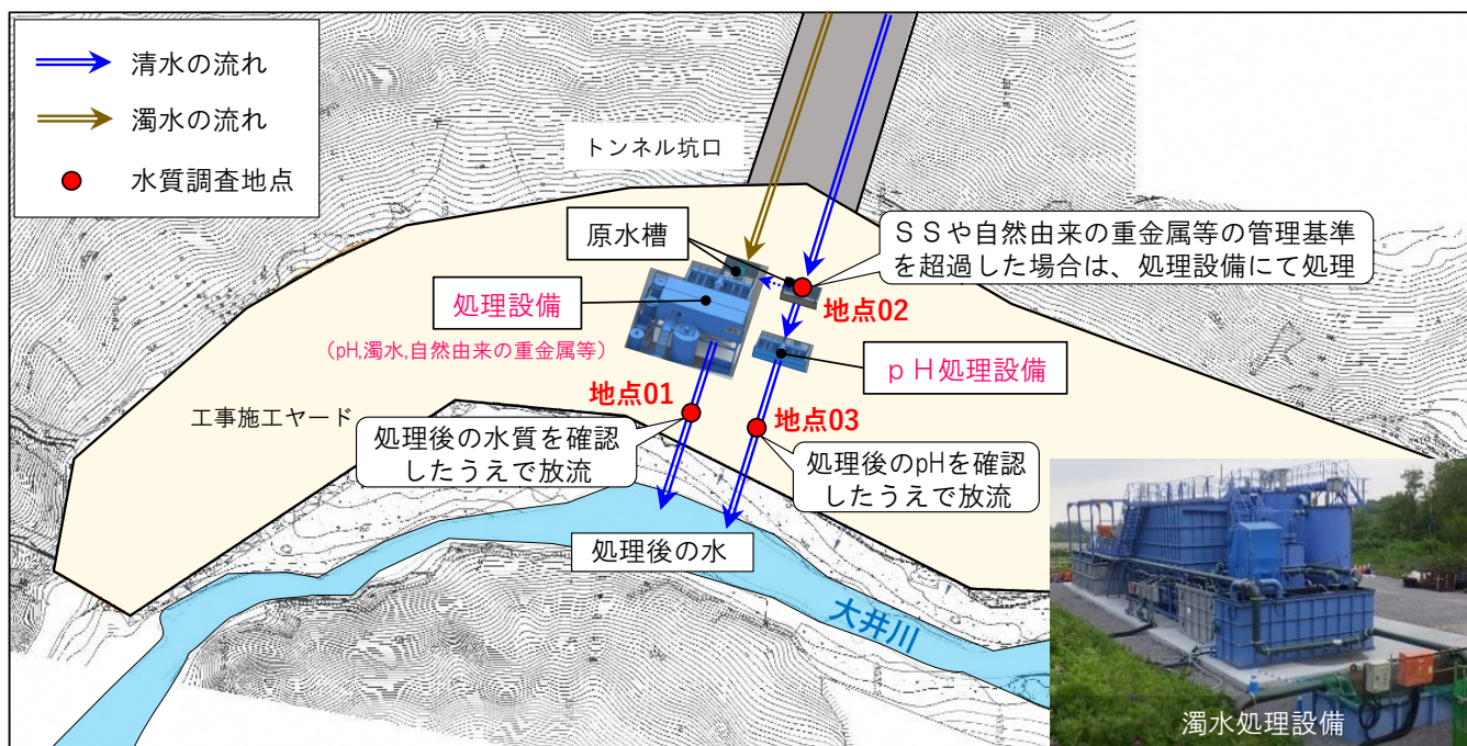
図 2 工事施工ヤードにおけるトンネル湧水等の処理の流れ（イメージ）
