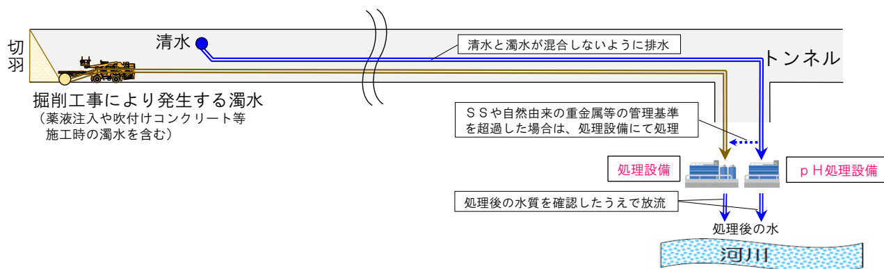
図 1 トンネル湧水等の清濁分離（イメージ）
