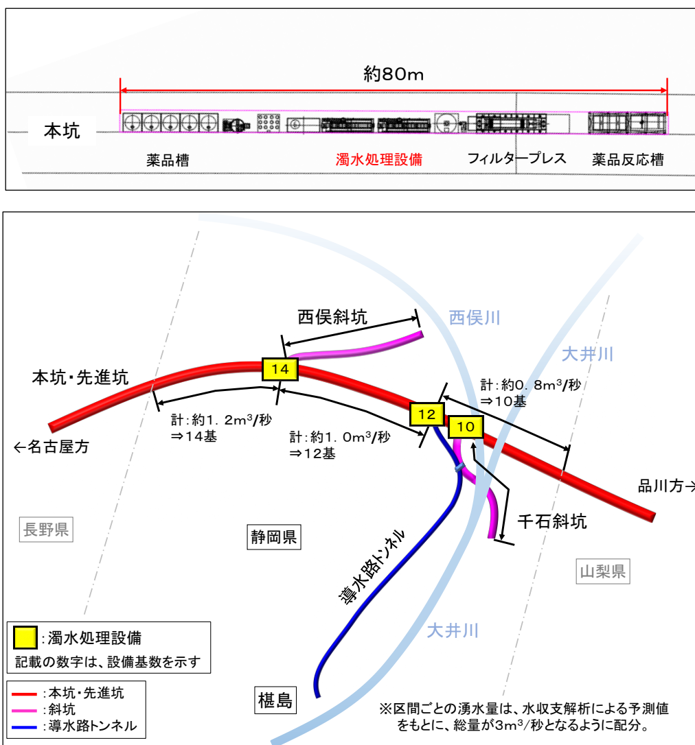
図 3 濁水処理設備の配置計画（仮に 3 \text{ m}^3/\text{秒} の濁水が発生した場合）
