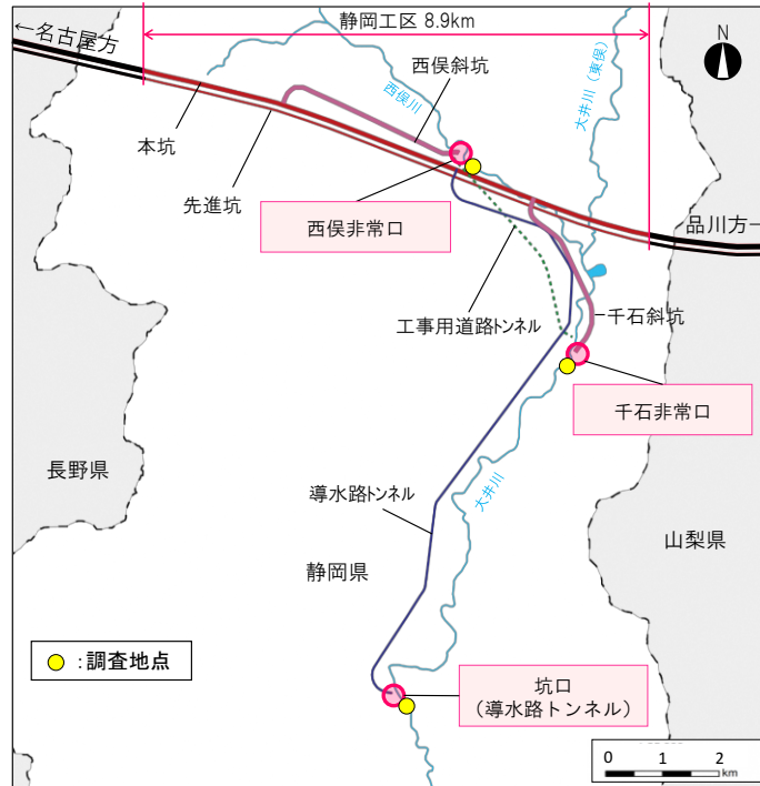
図 20 河川の水質・水温調査地点（トンネル湧水等の放流先河川の確認）
