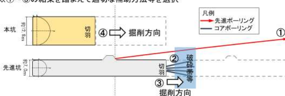
図 46 先進坑等の掘削手順
