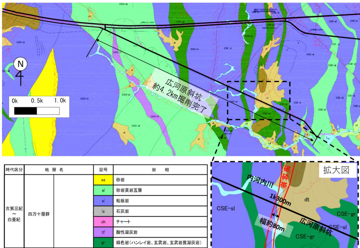
図 50 地質平面図
