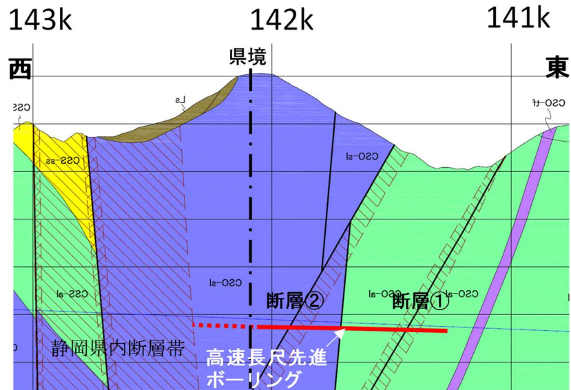
図 25 地質縦断図
