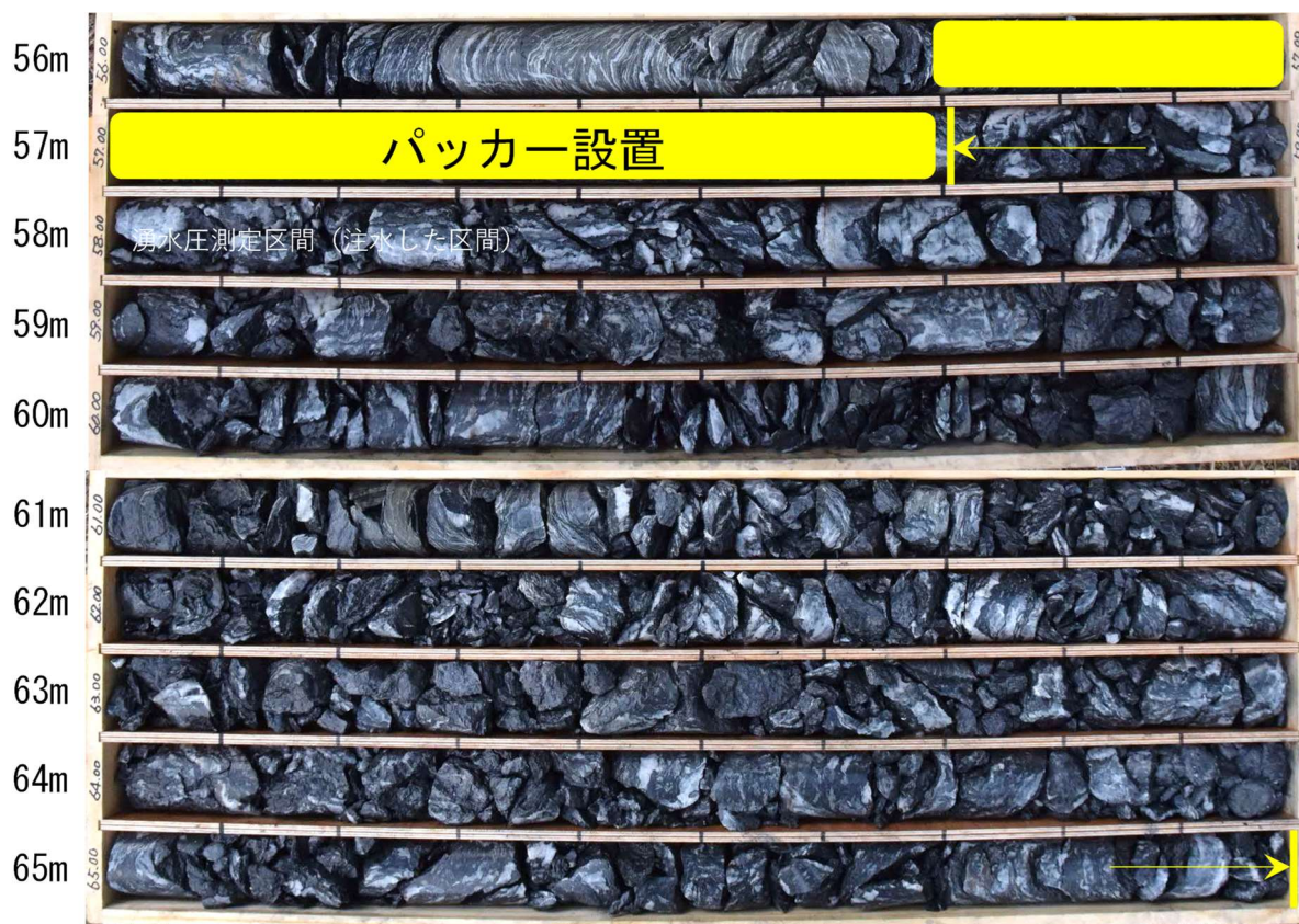
写真 5 孔内湧水圧測定 No. 1 (42.0m~50.2m) コア写真
