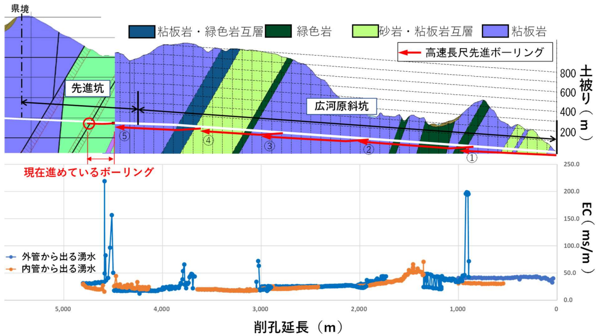
図 6 2 山梨県内の高速長尺先進ボーリング（広河原斜坑・先進坑）湧水の電気伝導度
