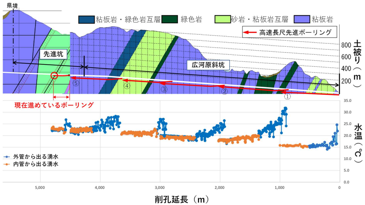
図 6 1 山梨県内の高速長尺先進ボーリング（広河原斜坑・先進坑）湧水の水温
