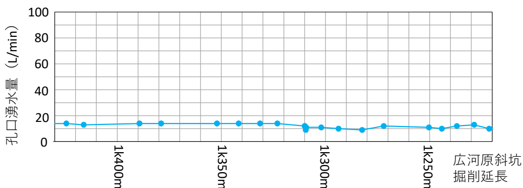
図 5 2 高速長尺先進ボーリング（広河原斜坑 0k850m～）の孔口湧水量
