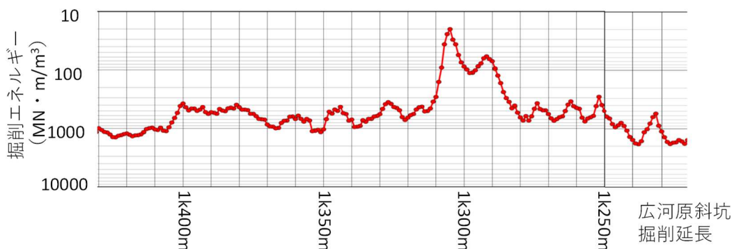
図 5 1 高速長尺先進ボーリング（広河原斜坑 0k850m～）の掘削エネルギー
