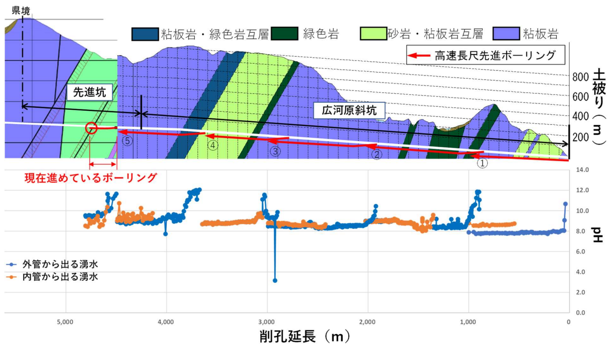
図 6 3 山梨県内の高速長尺先進ボーリング（広河原斜坑・先進坑）湧水の pH
