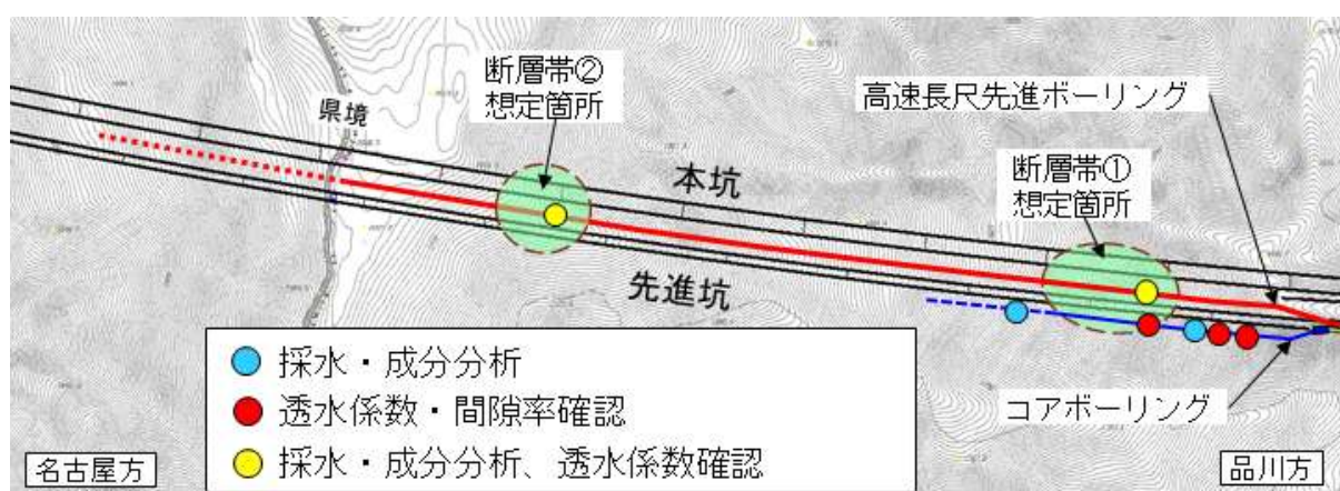
図 6 0 測定地点
