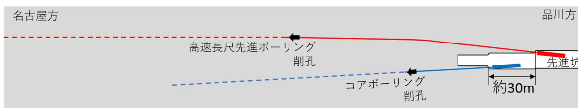
図 21 高速長尺先進ボーリングとコアボーリングの平面イメージ図
