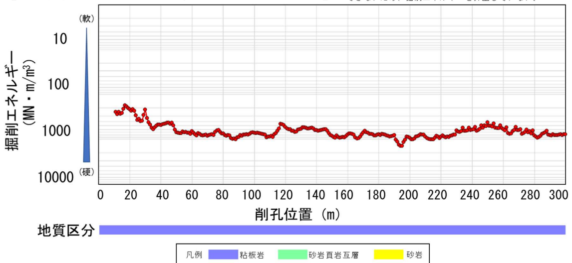
図 28 掘削エネルギー係数（孔口から300mまで）
