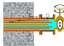
図 3 6 止水の手順
