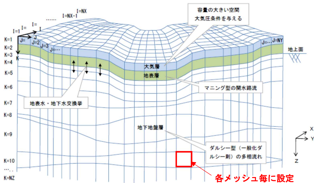
図 17 水収支解析モデル（静岡市モデル）
