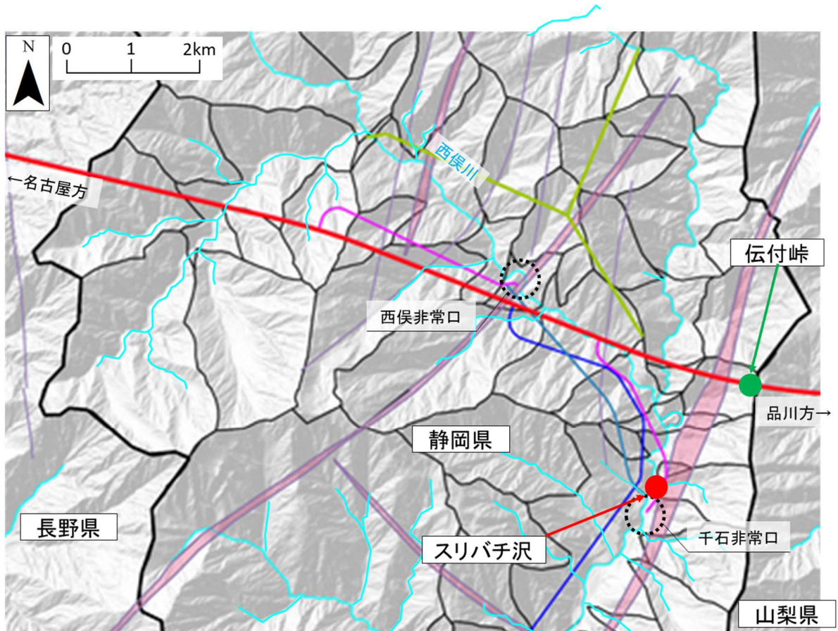
図 3 5 沢流量の測定の実施箇所
