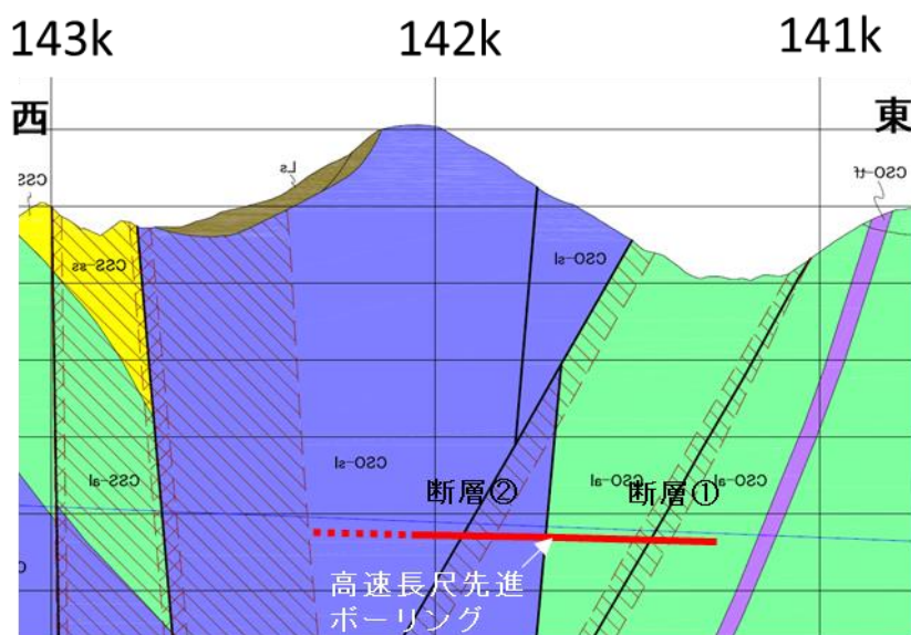
図 9 地質縦断図
