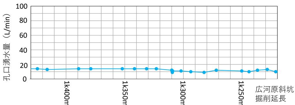
図 4 8 高速長尺先進ボーリング（広河原斜坑 0k850m～）の孔口湧水量
