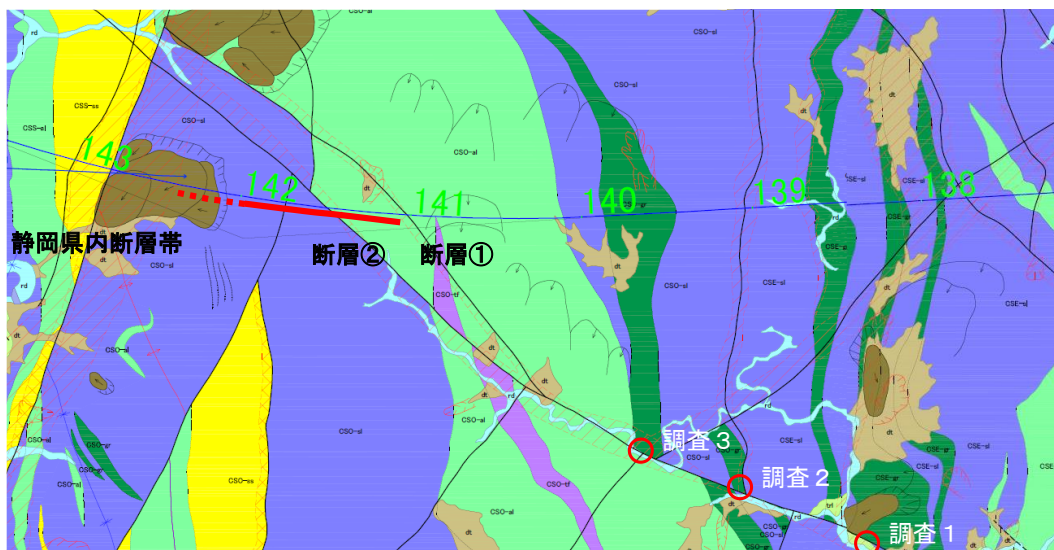
図 24 地質平面図
