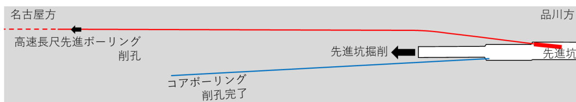
図 4 4 ボーリング調査と先進坑の平面イメージ図
