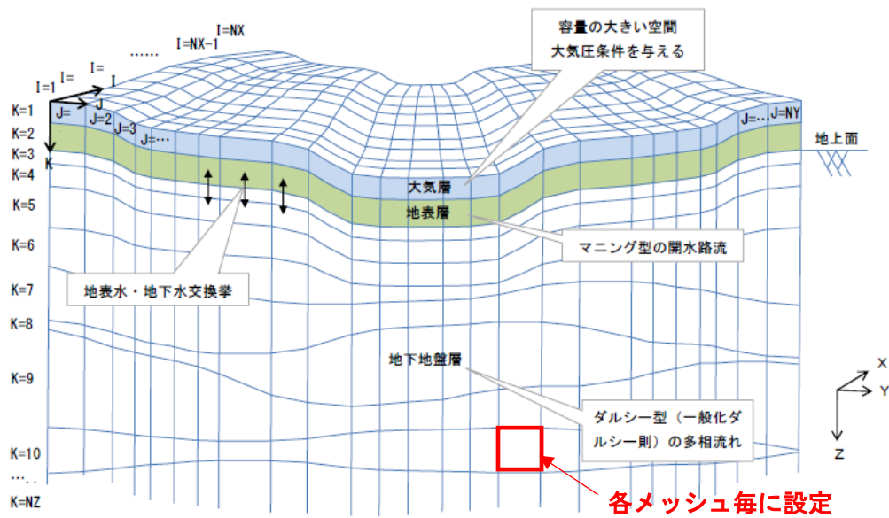
図 16 水収支解析モデル（静岡市モデル）
