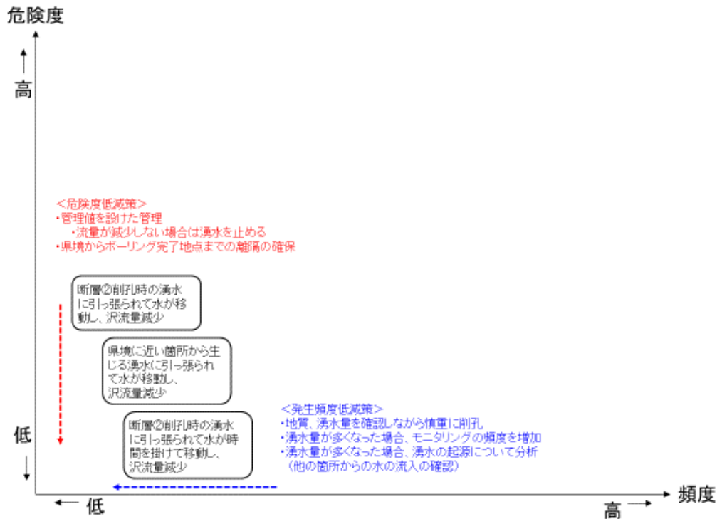
図 30 ボーリングに伴う湧水の発生に関わるリスクマップ
