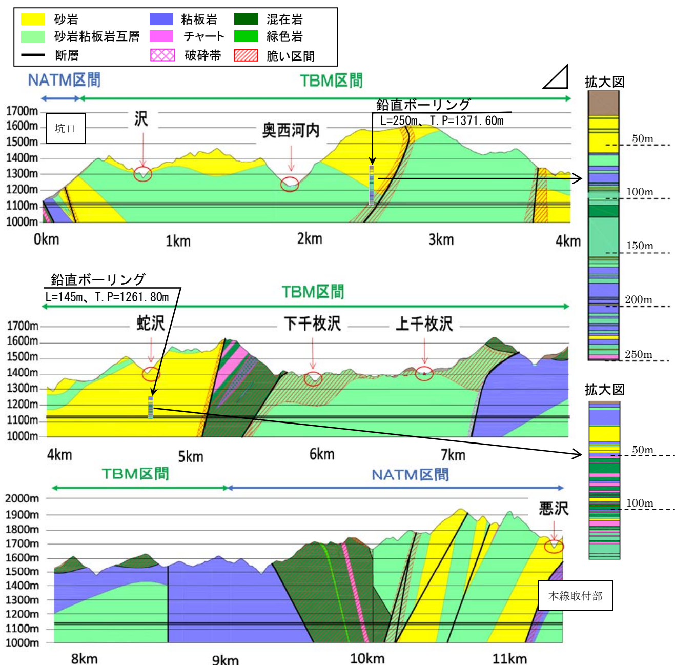
図 5.18 導水路トンネル 縦断図
