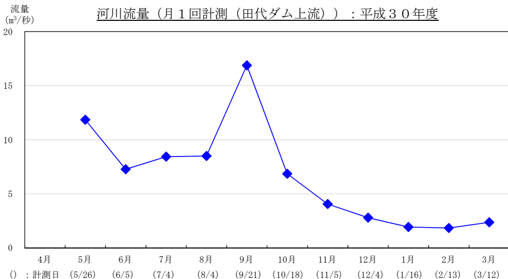
図 2-11 上流域の地下水位、河川流量調査結果(田代付近、平成30年度)
