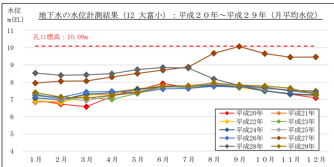
図 2-2 5 地下水の水位計測結果 (月平均水位) : 12 大富小 (焼津市中根新田)
