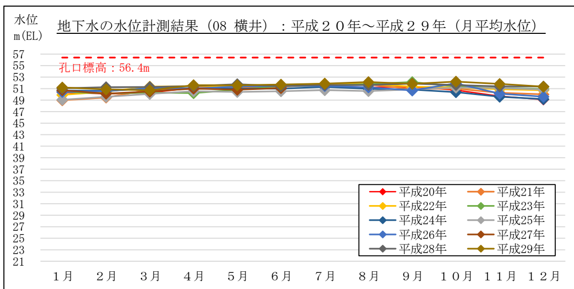
図 2-21 地下水の水位計測結果 (月平均水位) : 08 横井 (島田市横井)
