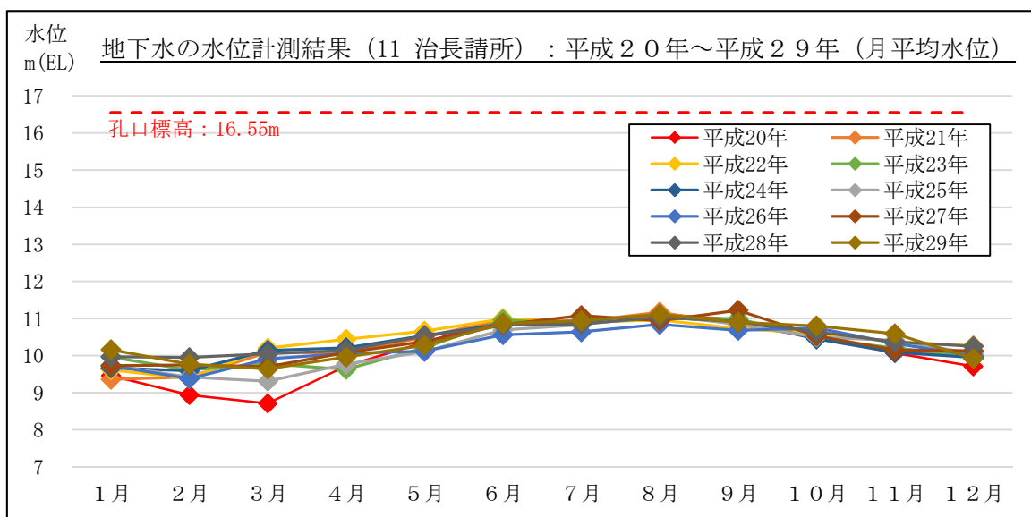
図 2-2 4 地下水の水位計測結果 (月平均水位) : 11 治長請所 (焼津市治長請所)
