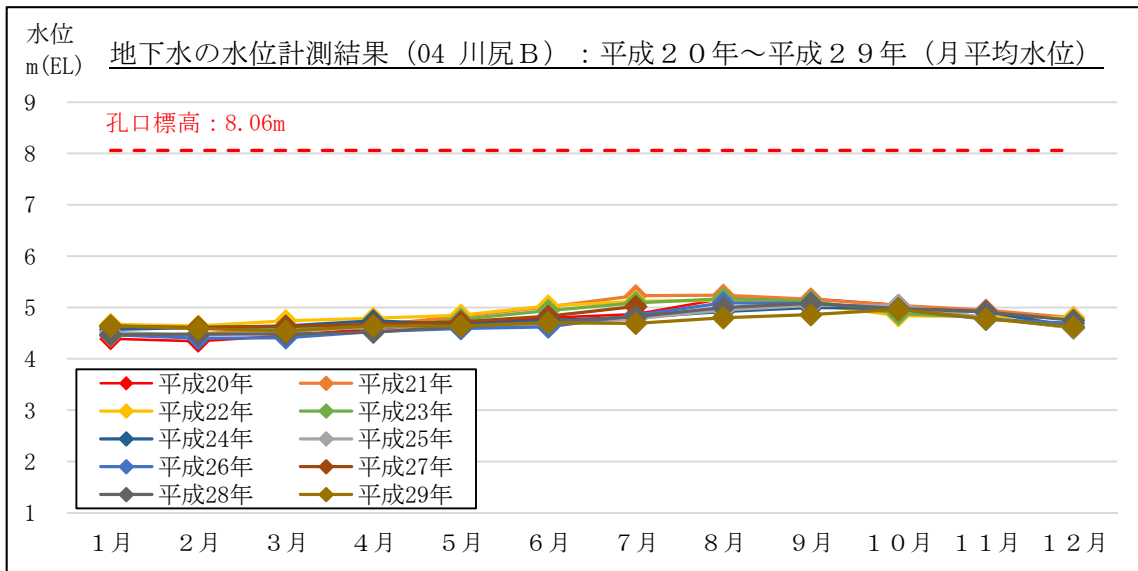
図 2-17 地下水の水位計測結果 (月平均水位) : 04 川尻B (吉田町川尻)
