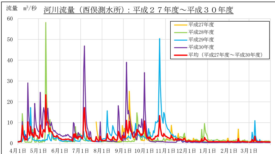
図 2-3 流量計測結果（常時計測：西俣測水所）
