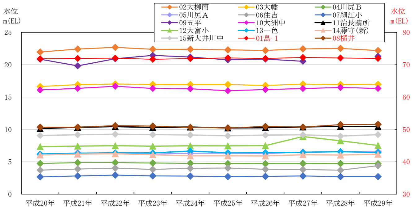
図 2-13 地下水の水位計測結果 (年平均水位)
