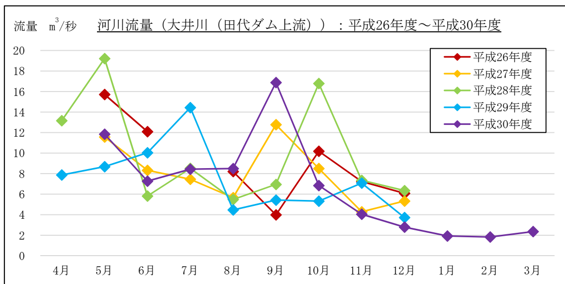
図 2-4 流量計測結果（月1回計測：田代ダム上流）
