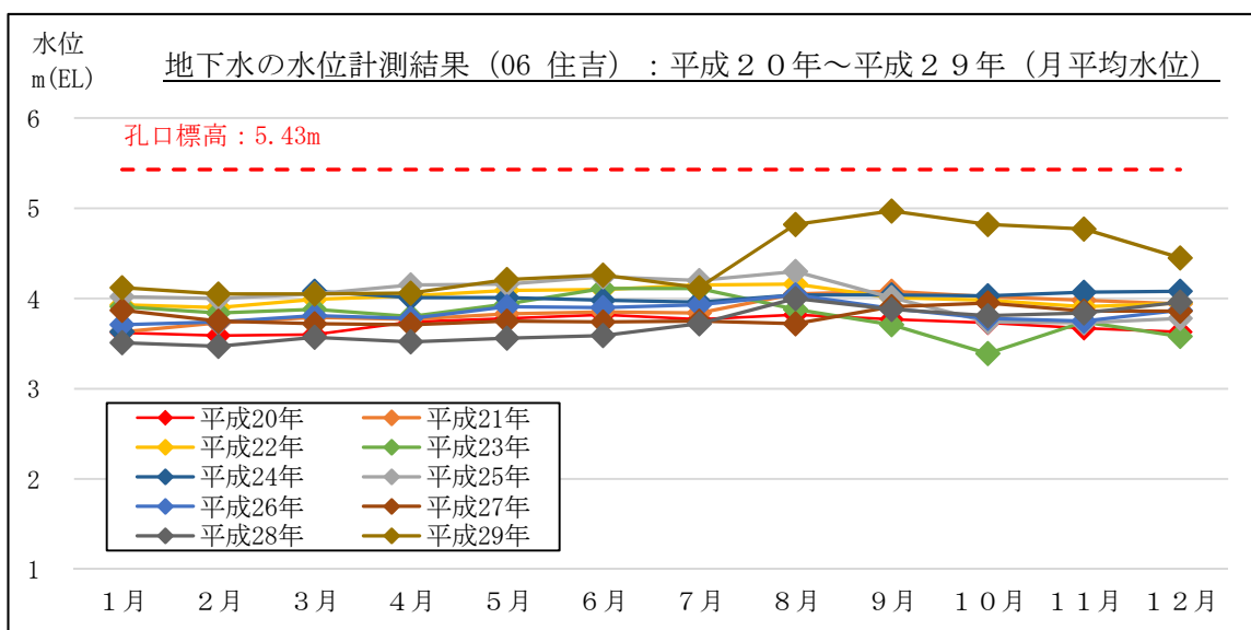
図 2-19 地下水の水位計測結果 (月平均水位) : 06 住吉 (吉田町住吉)
