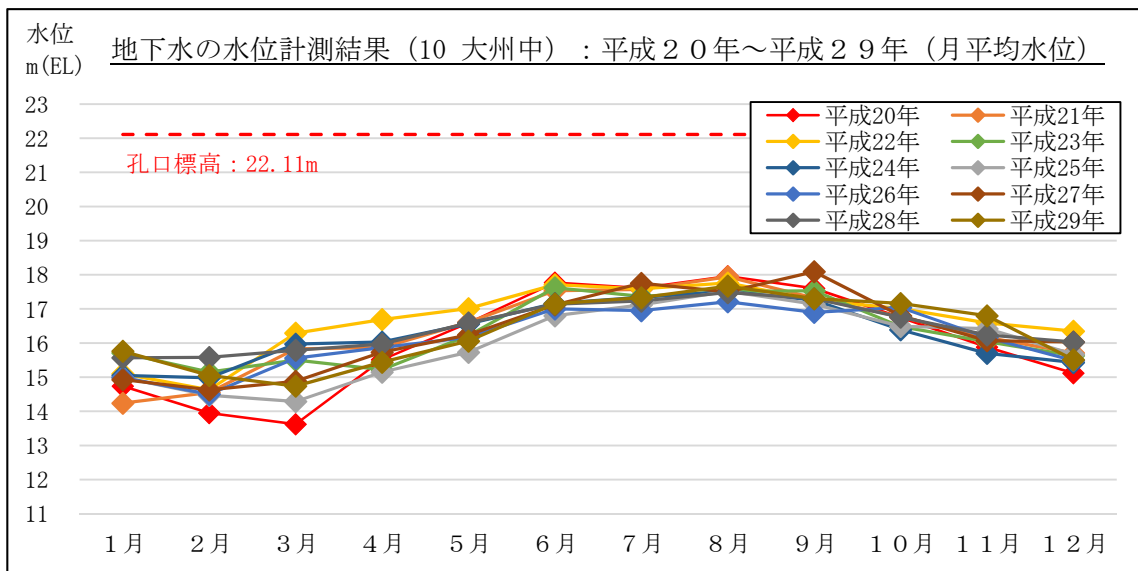
図 2-2 3 地下水の水位計測結果 (月平均水位) : 10 大州中 (藤枝市弥左工門)
