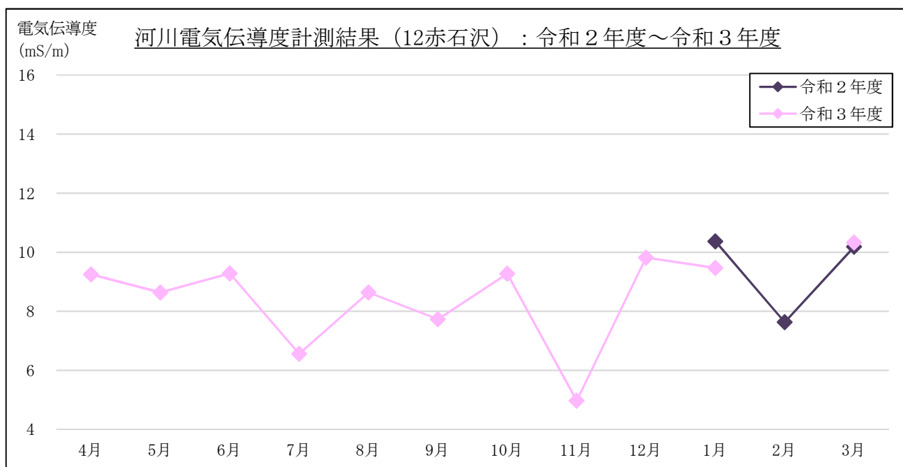
図 2-1-9(8) 電気伝導度計測結果 (流量 (月1回計測箇所)) : 12 赤石沢
