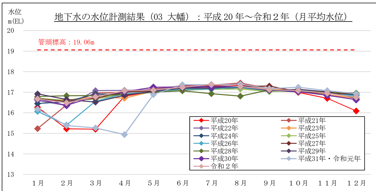
図 3-2-2(5) 地下水の水位計測結果 (月平均水位) : 03 大幡 (吉田町大幡)
