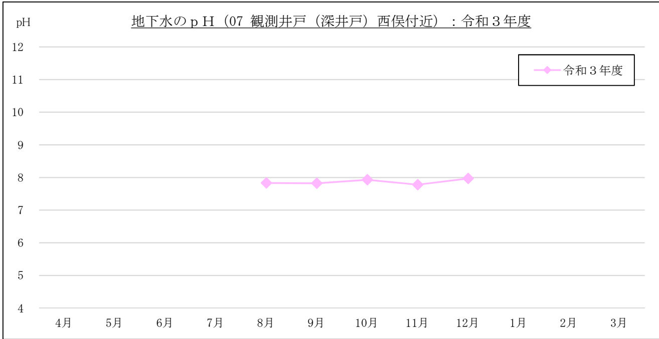
図 3-1-4(9) 地下水のpH計測結果 : 07 観測井戸 (深井戸) 西俣付近
