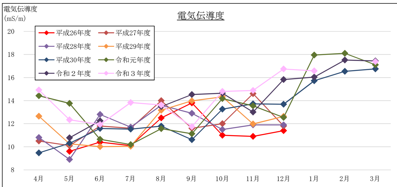
图 2-1-5(3) 電気伝導度計測結果 (流量 (常時計測箇所)) : 03 木賊測水所付近
