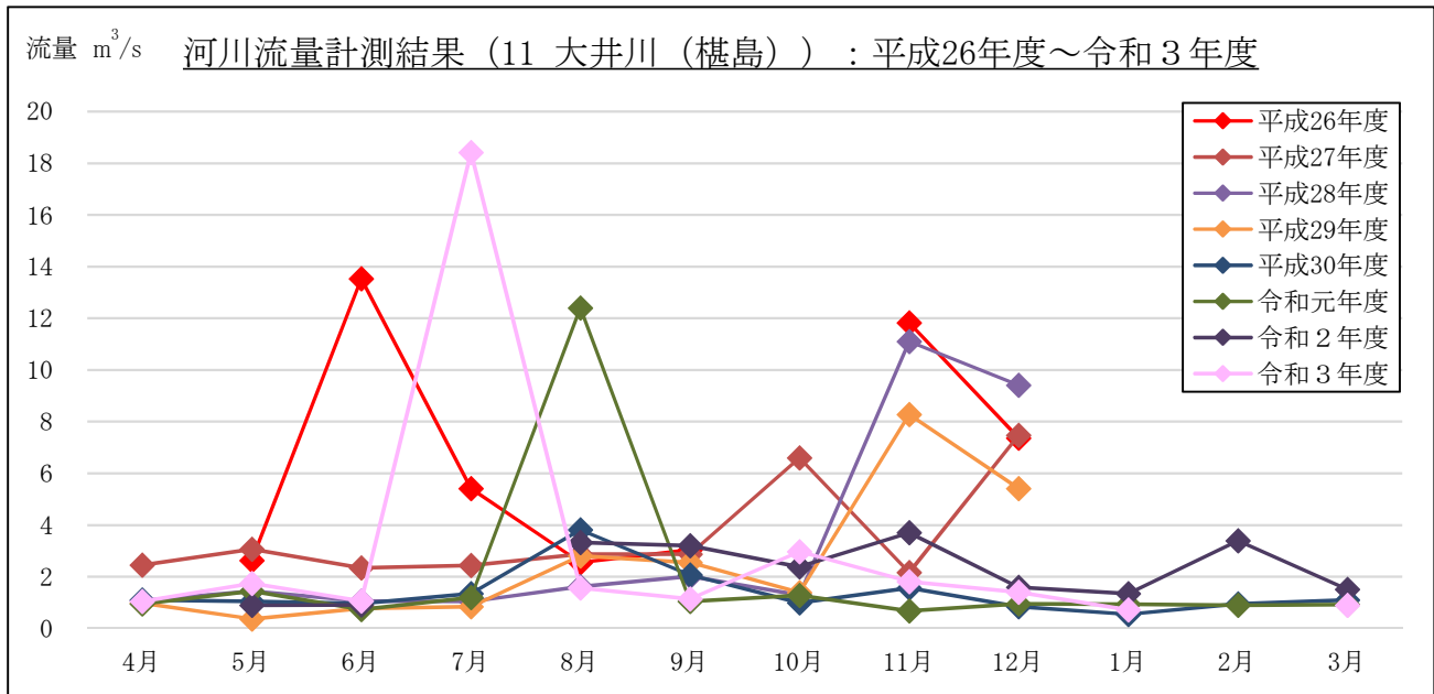
図 2-1-6(7) 流量計測結果（流量（月1回計測箇所））：11 大井川（樺島）
