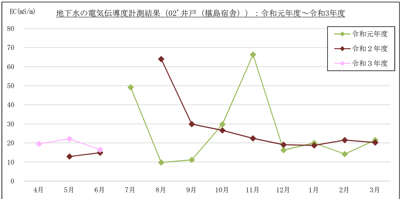
図 3-1-5(3) 地下水の電気伝導度計測結果 : 02' 井戸 (樫島宿舎)
