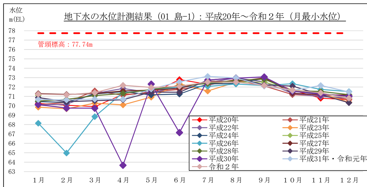
図 3-2-2(2) 地下水の水位計測結果 (月最小水位) : 01 島-1 (島田市島)
