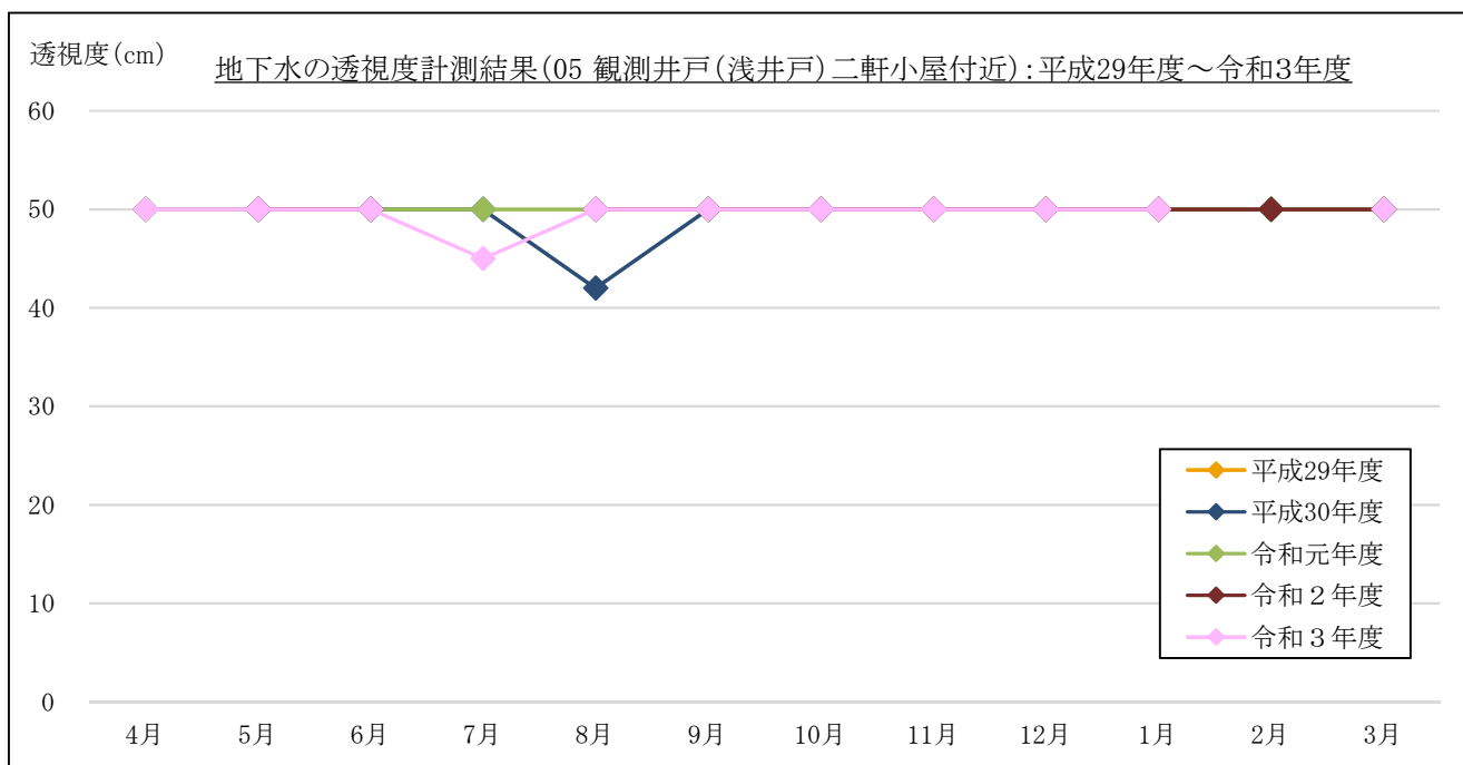
図 3-1-6(7) 地下水の透視度計測結果 : 05 観測井戸 (浅井戸) 二軒小屋付近
