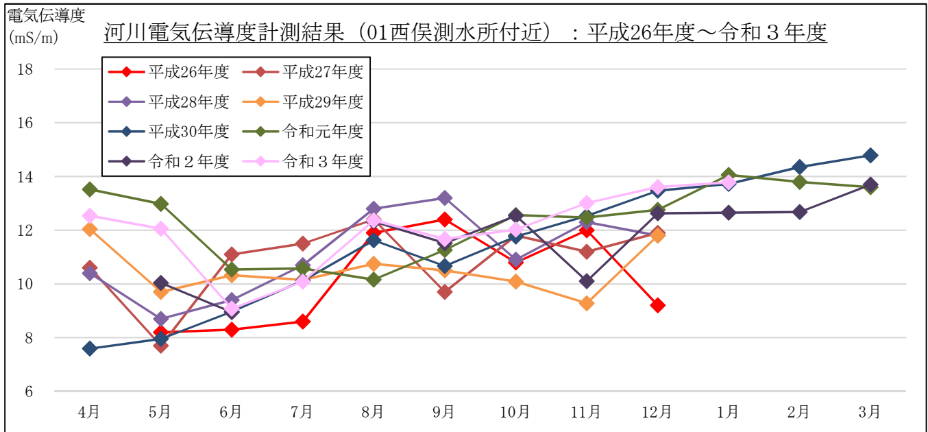
図 2-1-5(1) 電気伝導度計測結果 (流量 (常時計測箇所)) : 01 西俣測水所付近
