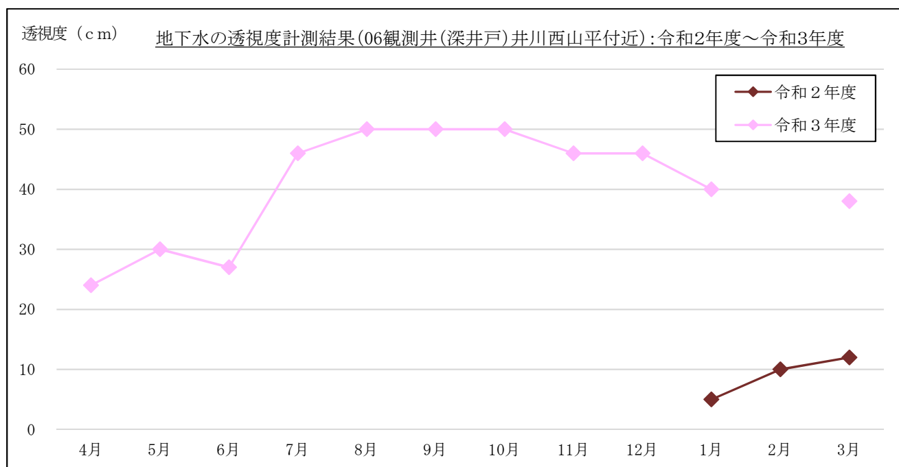
図 3-1-6(8) 地下水の透視度計測結果 : 06 観測井戸 (深井戸) 井川西山平付近
