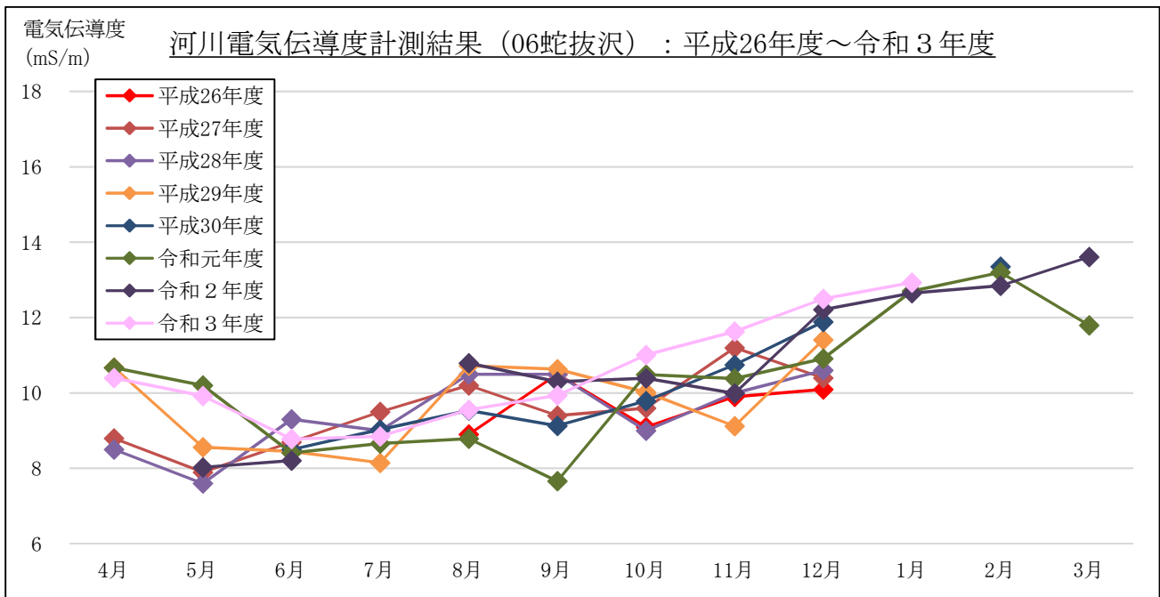
図 2-1-9(2) 電気伝導度計測結果 (流量 (月1回計測箇所)) : 06 蛇抜沢
