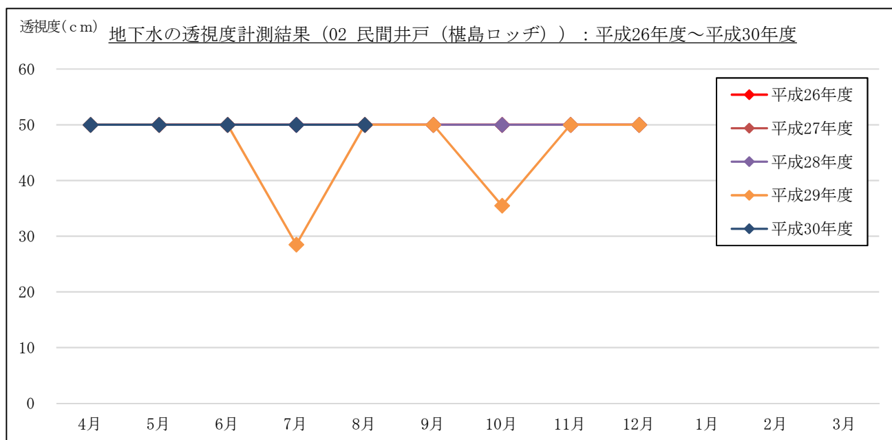
図 3-1-6(2) 地下水の透視度計測結果 : 02 民間井戸 (榎島ロッヂ)
