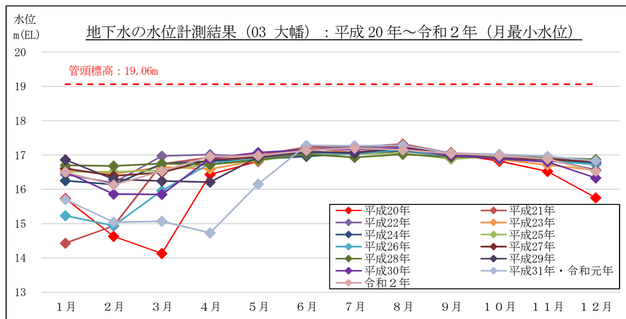
図 3-2-2(6) 地下水の水位計測結果 (月最小水位) : 03 大幡 (吉田町大幡)
