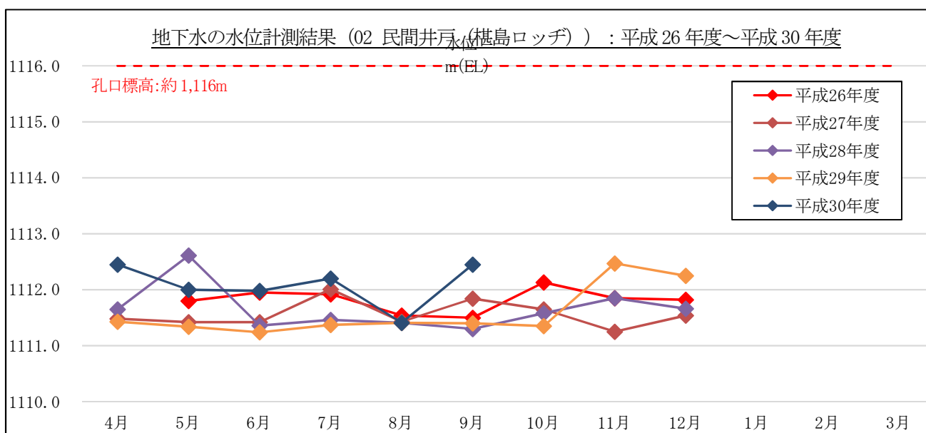
図 3-1-2(2) 地下水の水位計測結果 (月 1 回計測) : 02 民間井戸 (榎島ロッヂ)
