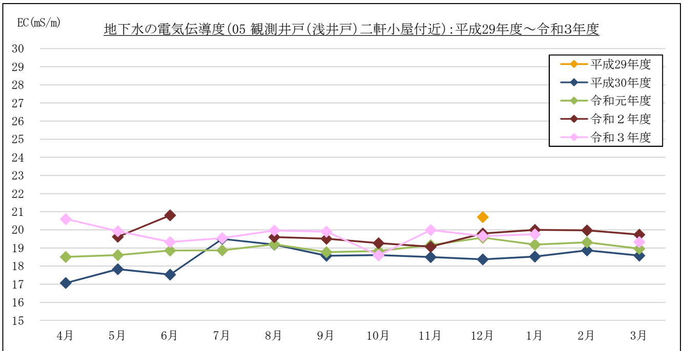
図 3-1-5(7) 地下水の電気伝導度計測結果 : 05 観測井戸 (浅井戸) 二軒小屋付近
