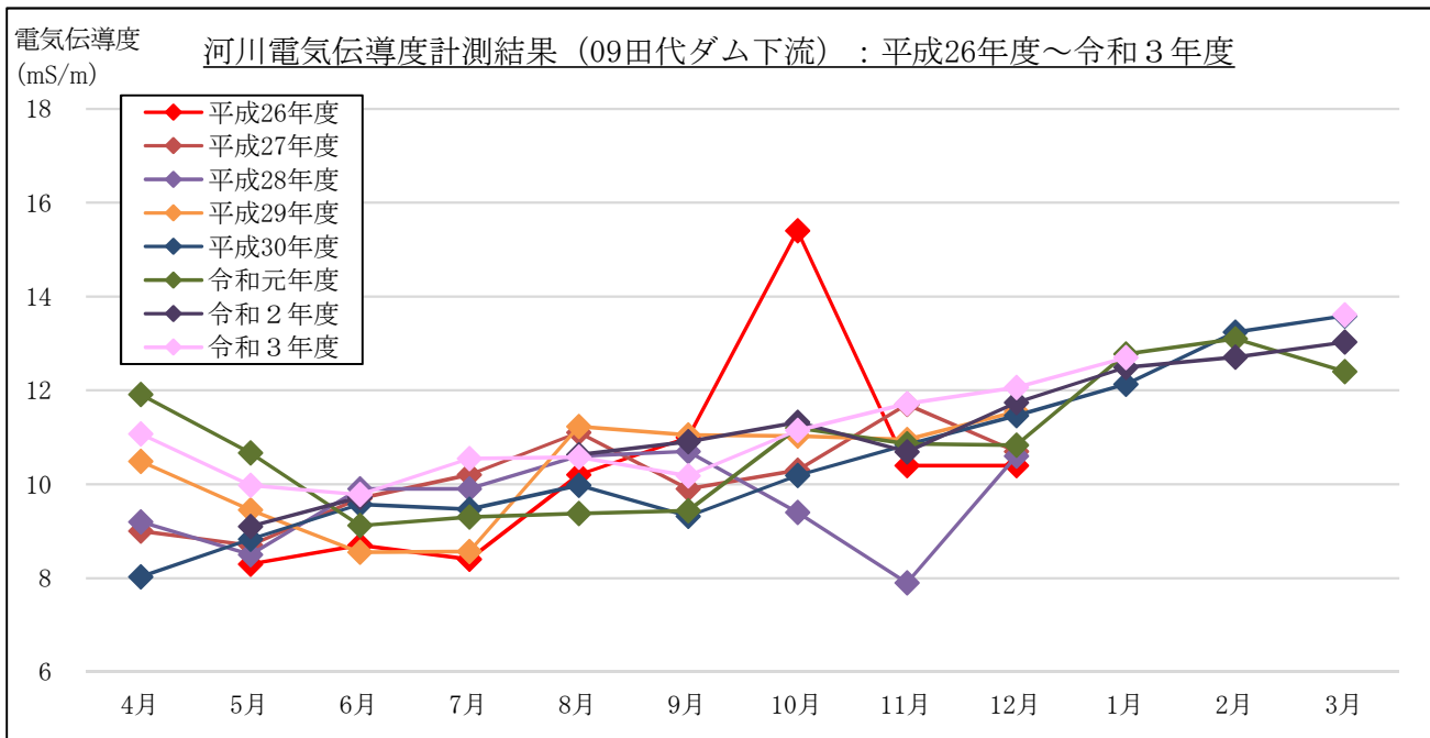
図 2-1-9(5) 電気伝導度計測結果 (流量 (月1回計測箇所)) : 09 大井川 (田代ダム下流)
