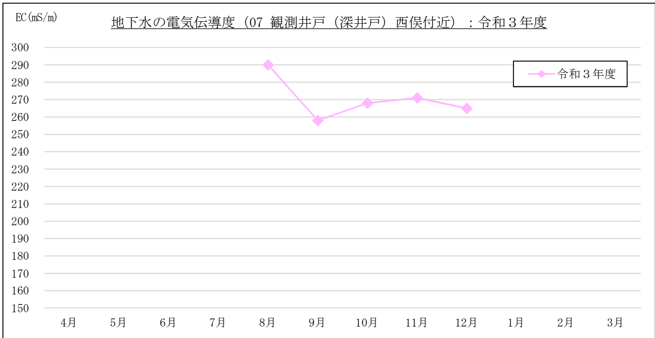
図 3-1-5(9) 地下水の電気伝導度計測結果 : 07 観測井戸 (深井戸) 西俣付近
