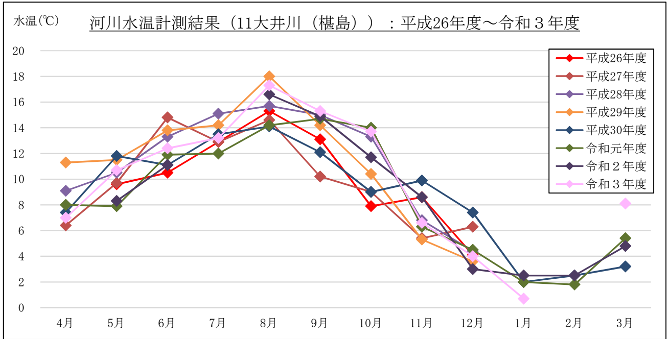
図 2-1-7(7) 水温計測結果 (流量 (月1回計測箇所)) : 11 大井川 (榎島)
