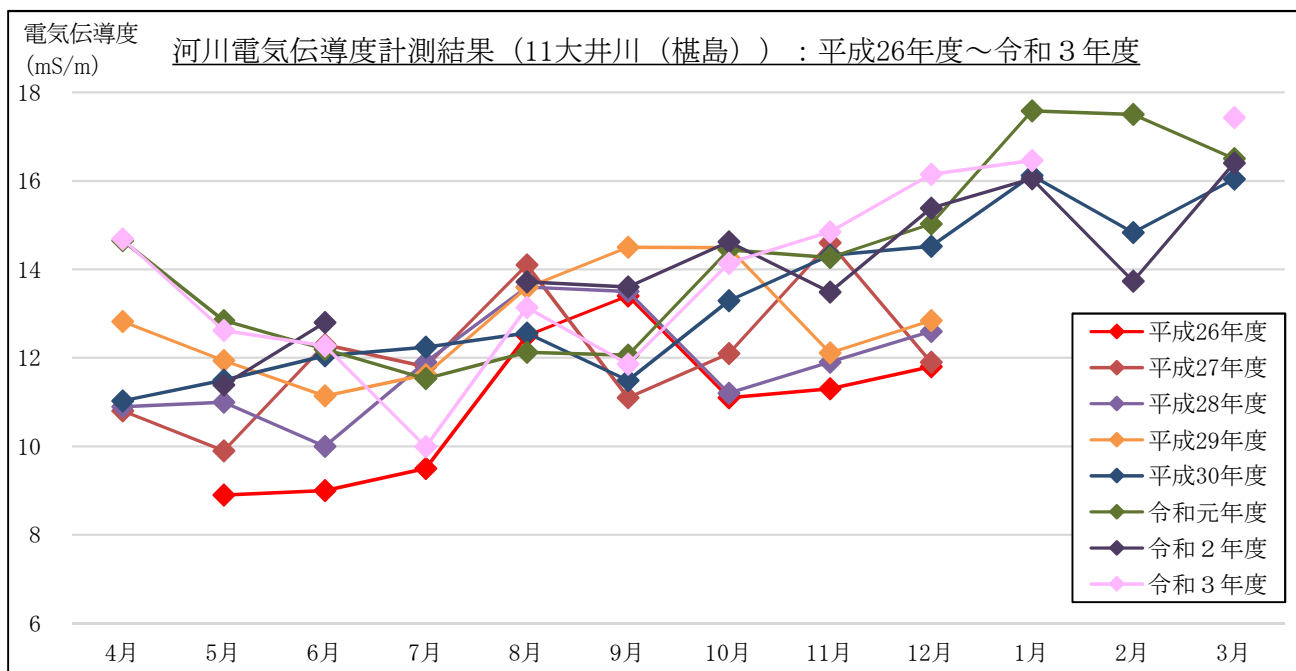
図 2-1-9(7) 電気伝導度計測結果 (流量 (月1回計測箇所)) : 11 大井川 (樫島)
