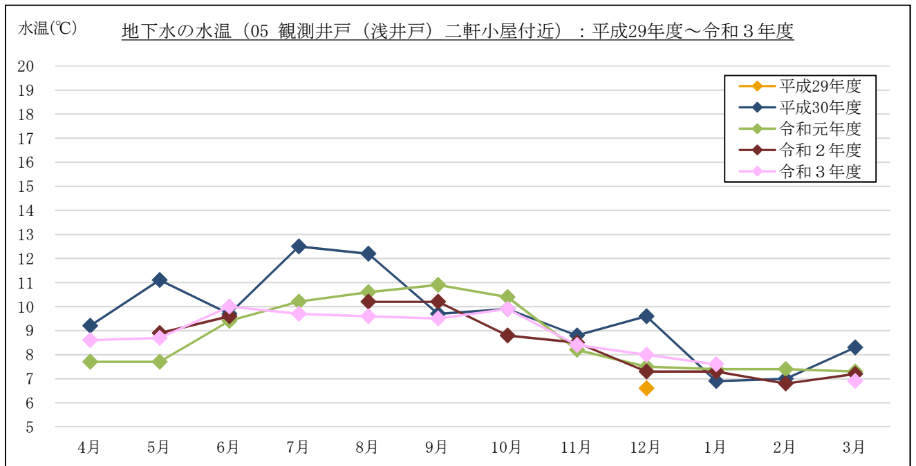
図 3-1-3(7) 地下水の水温計測結果 : 05 観測井戸 (浅井戸) 二軒小屋付近
