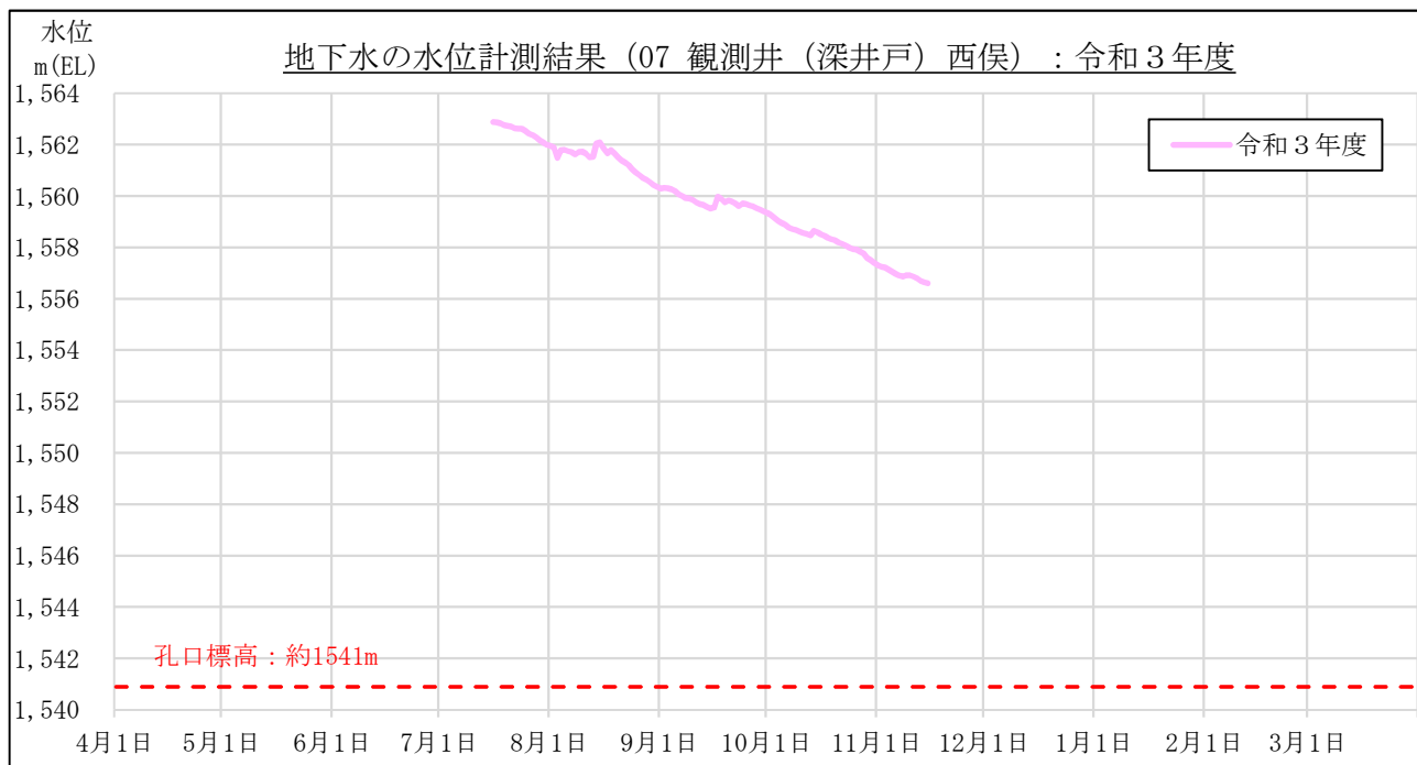
図 3-1-2(9) 地下水の水位計測結果 (常時計測) : 07 観測井戸 (深井戸) 西俣付近
