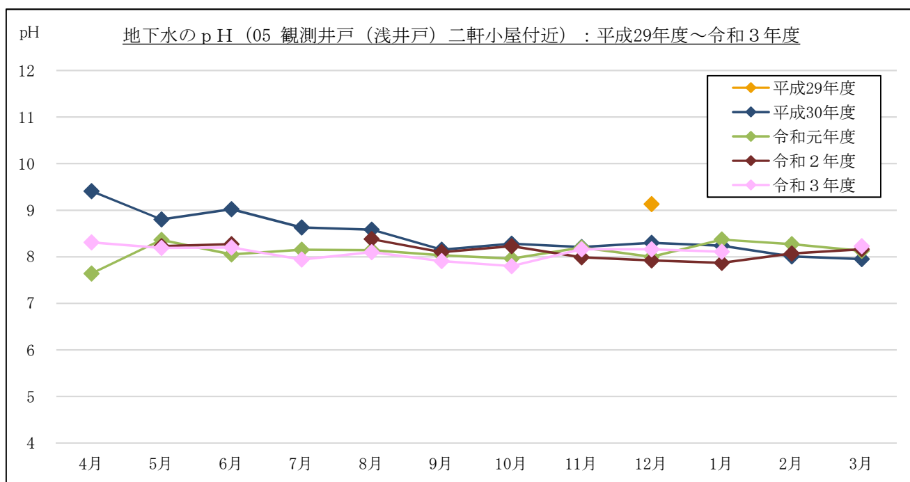
図 3-1-4(7) 地下水のpH計測結果 : 05 観測井戸 (浅井戸) 二軒小屋付近
