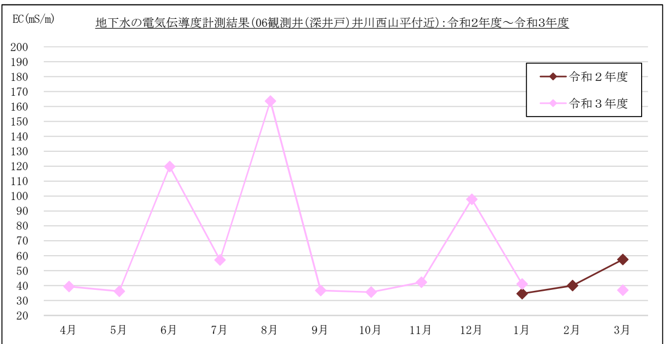
図 3-1-5 図 3-1-2(8) 地下水の電気伝導度計測結果 : 06 観測井戸 (深井戸) 井川西山平付近
