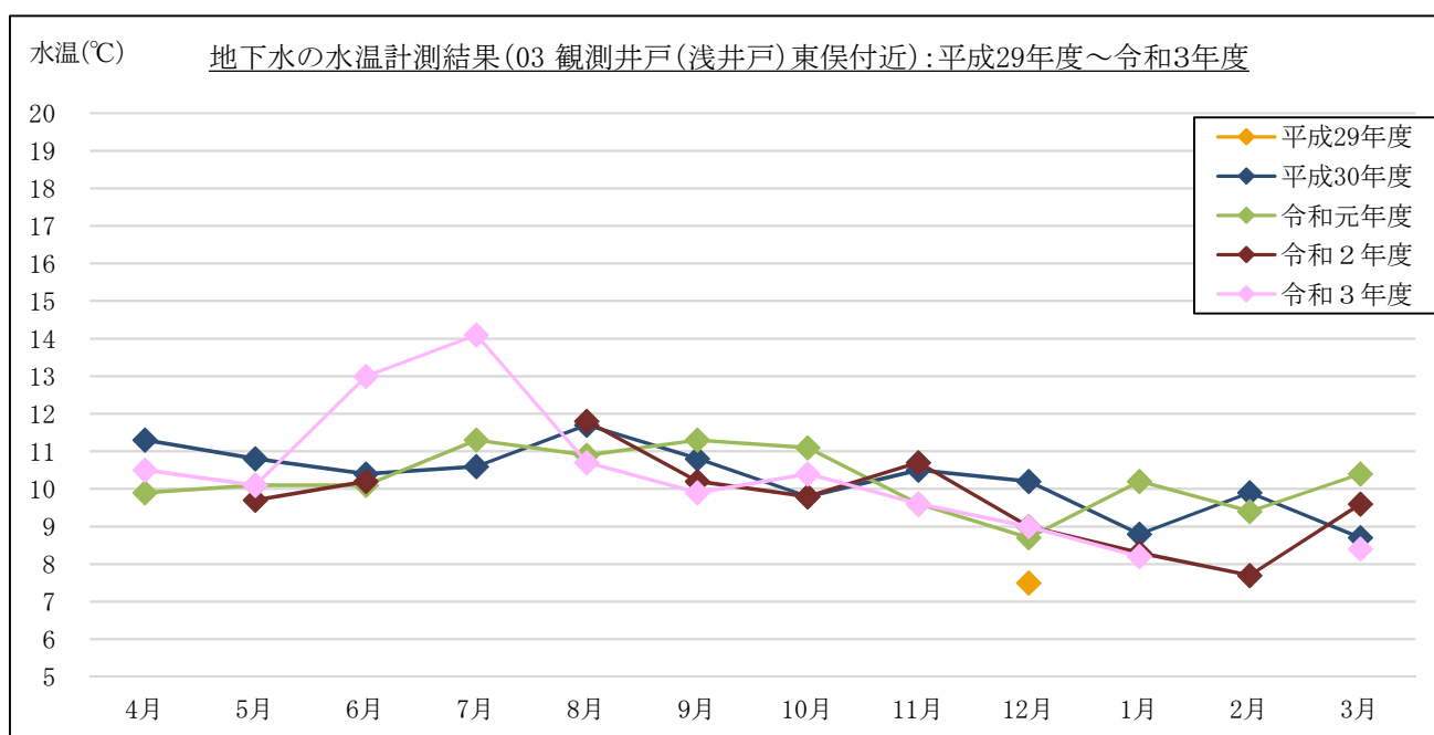
図 3-1-3(4) 地下水の水温計測結果 : 03 観測井戸 (浅井戸) 東俣付近
