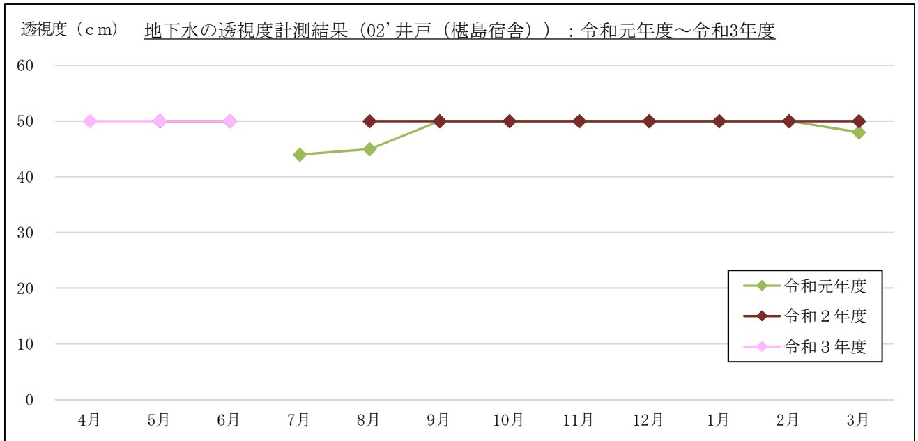
図 3-1-6(3) 地下水の透視度計測結果 : 02' 井戸 (榎島宿舎)
