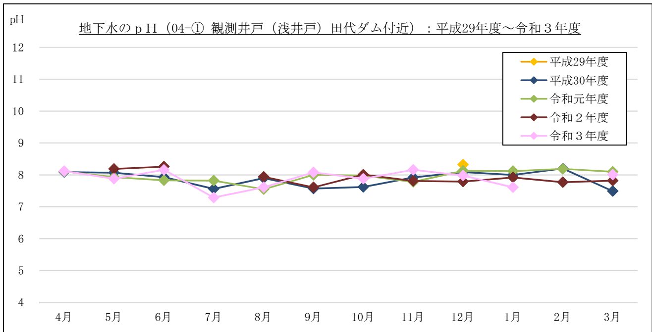
図 3-1-4(5) 地下水のpH計測結果 : 04-① 観測井戸 (浅井戸) 田代ダム付近
