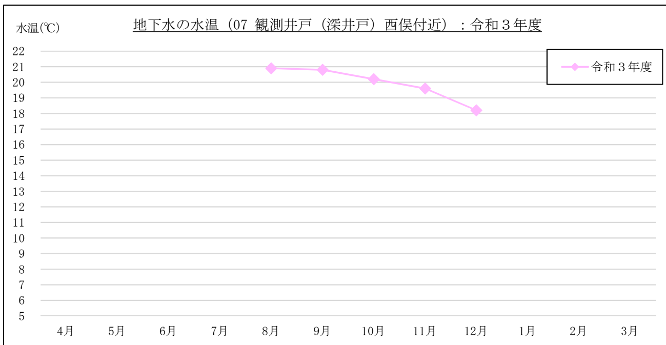
図 3-1-3(9) 地下水の水温計測結果 : 07 観測井戸 (深井戸) 西俣付近
