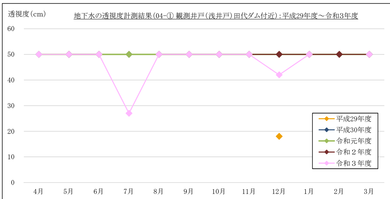
図 3-1-6(5) 地下水の透視度計測結果：04-① 観測井戸（浅井戸）田代ダム付近
