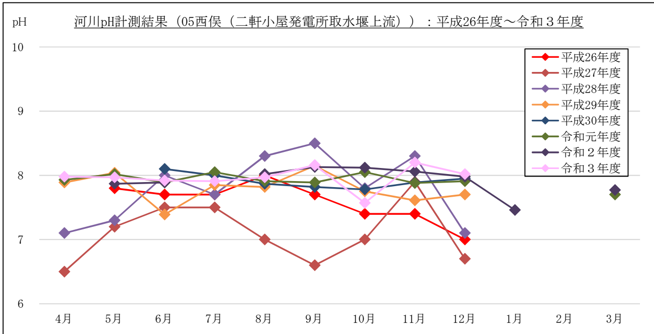
图 2-1-8(1) pH 計測結果 (流量 (月 1 回計測箇所)) : 05 西俣 (二軒小屋発電所取水堰上流)
