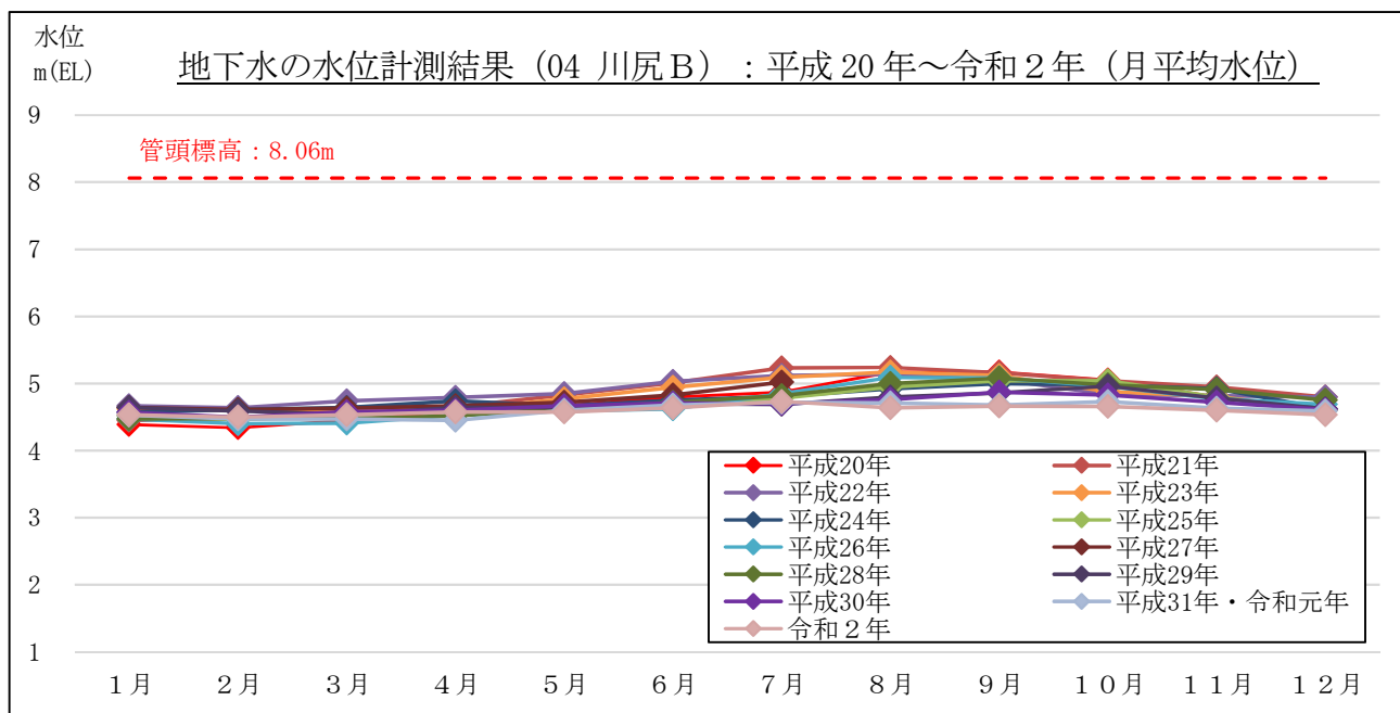
図 3-2-2(7) 地下水の水位計測結果 (月平均水位) : 04 川尻B (吉田町川尻)
