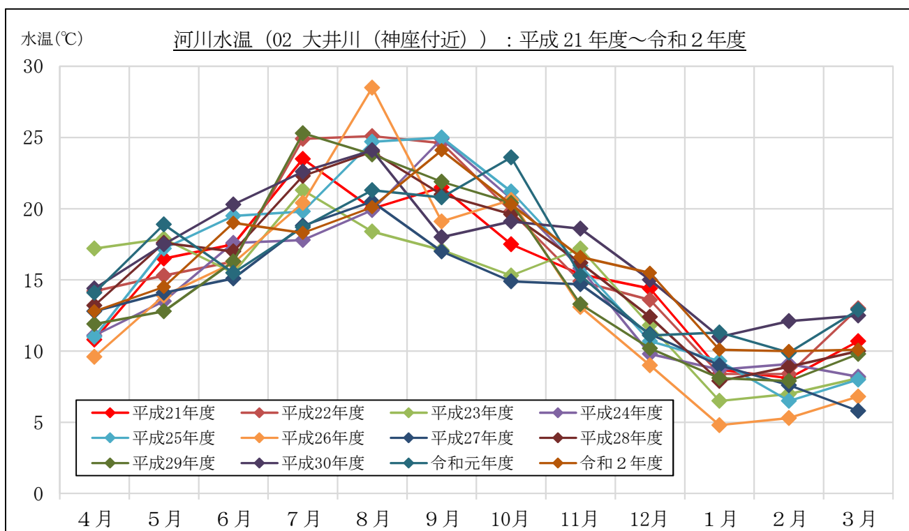
図 2-2-3(2) 水温計測結果 : 02 大井川 (神座付近)
