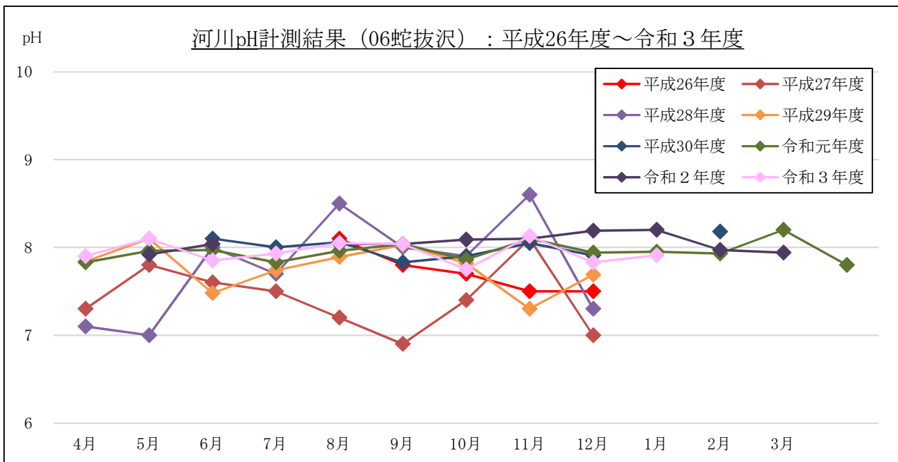
图 2-1-8(2) pH 計測結果 (流量 (月 1 回計測箇所)) : 06 蛇抜沢
