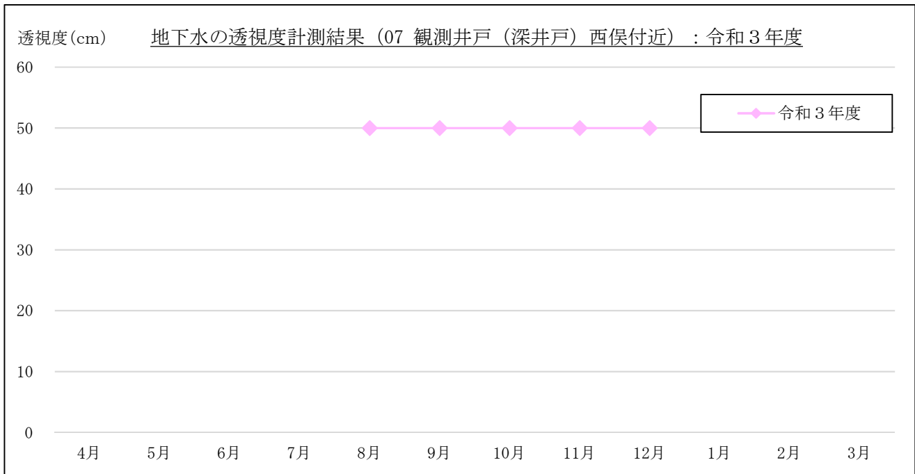
図 3-1-6(9) 地下水の透視度計測結果 : 07 観測井戸 (深井戸) 西俣付近
