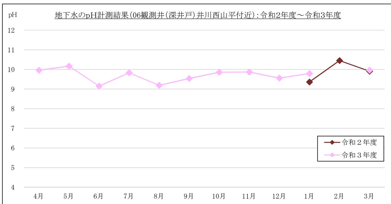
図 3-1-4(8) 地下水のpH計測結果 : 06 観測井戸 (深井戸) 井川西山平付近
