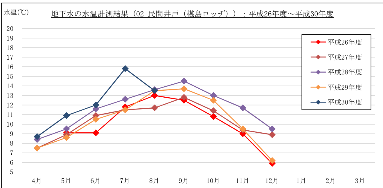
図 3-1-3(2) 地下水の水温計測結果 : 02 民間井戸 (樫島ロッヂ)
