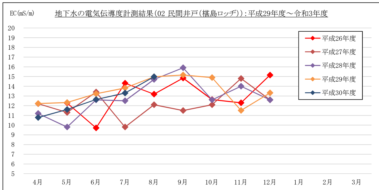
図 3-1-5(2) 地下水の電気伝導度計測結果 : 02 民間井戸 (樺島ロッヂ)
