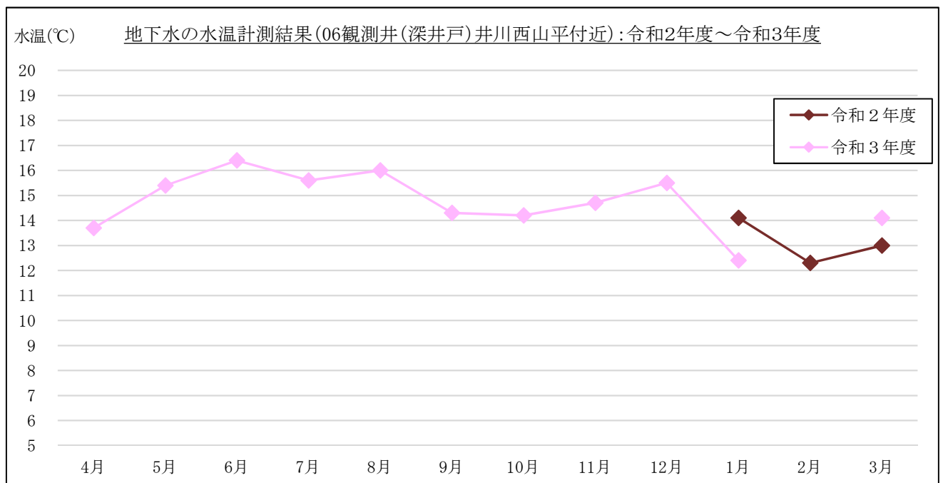
図 3-1-3(8) 地下水の水温計測結果 : 06 観測井戸 (深井戸) 井川西山平付近
