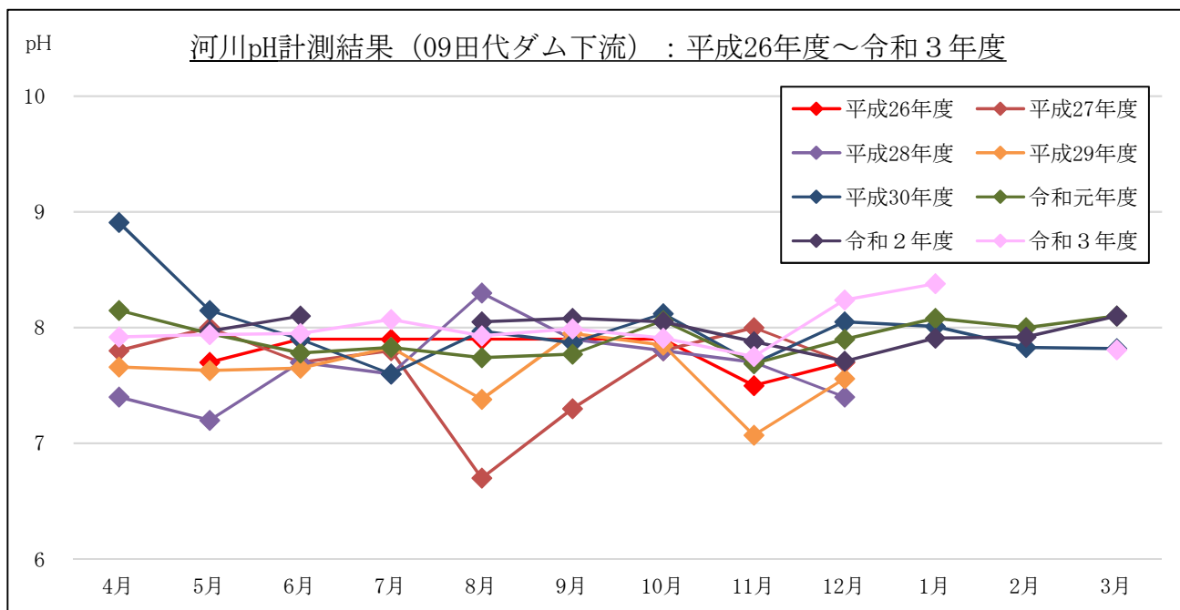
図 2-1-8(5) pH計測結果（流量（月1回計測箇所））：09 大井川（田代ダム下流）
