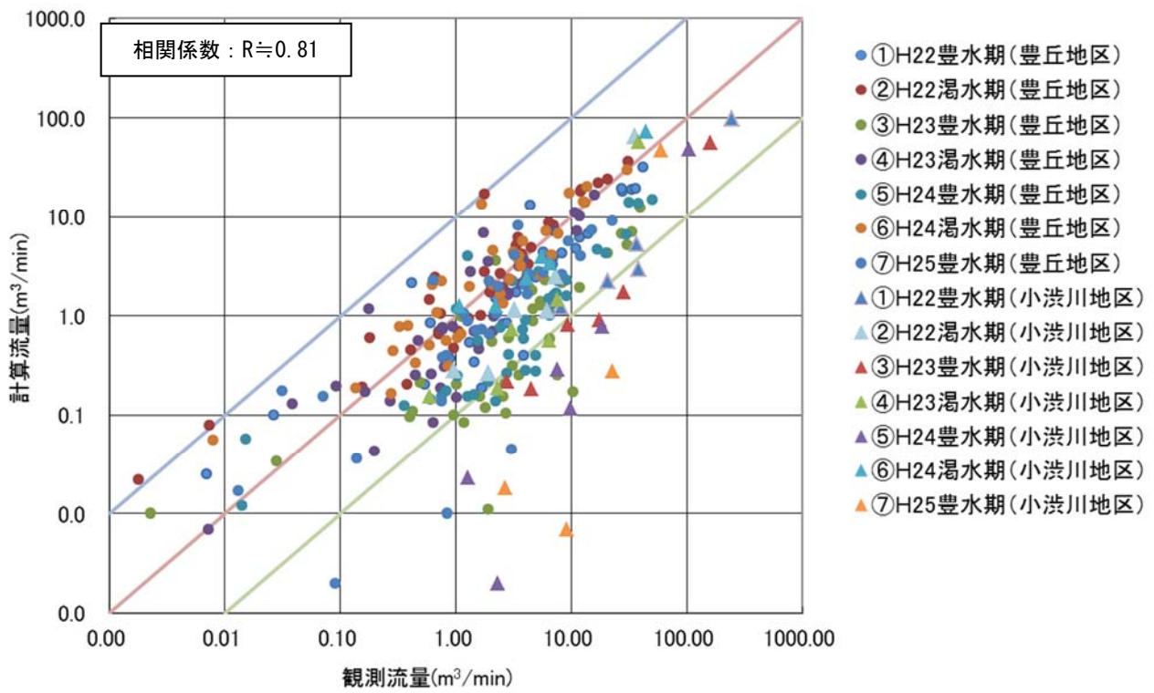
図 6 観測流量と計算流量の比較
