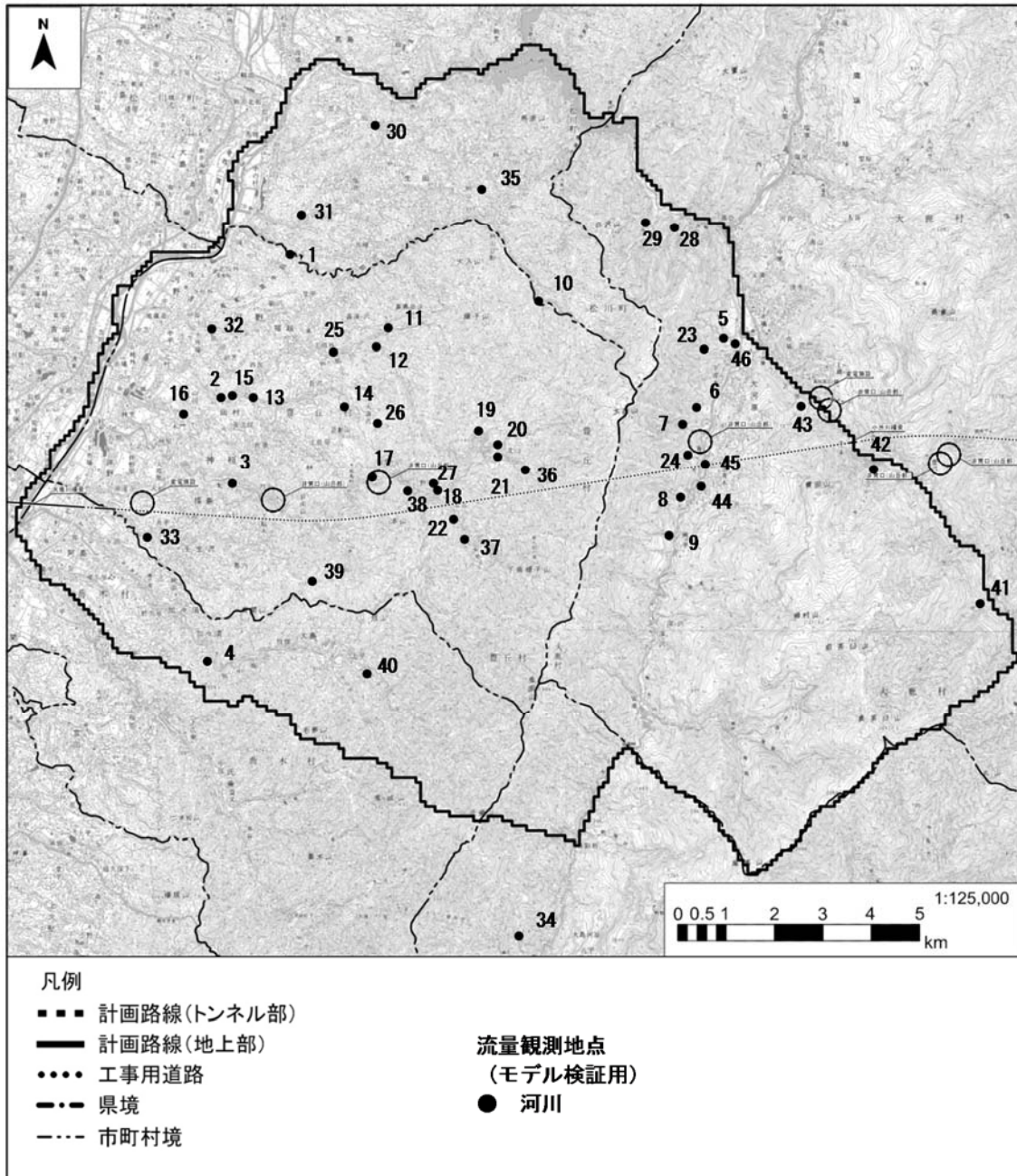
図5 検証に使用した流量観測地点
