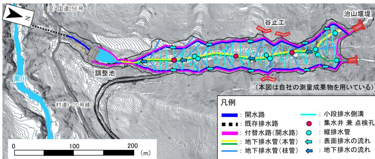
図 3-8 発生土置き場における排水計画図
