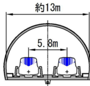
トンネルの標準的な断面図 (山岳トンネル)
