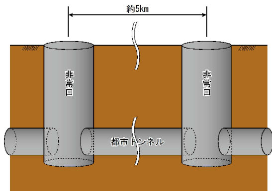
非常口（都市部）の概要
