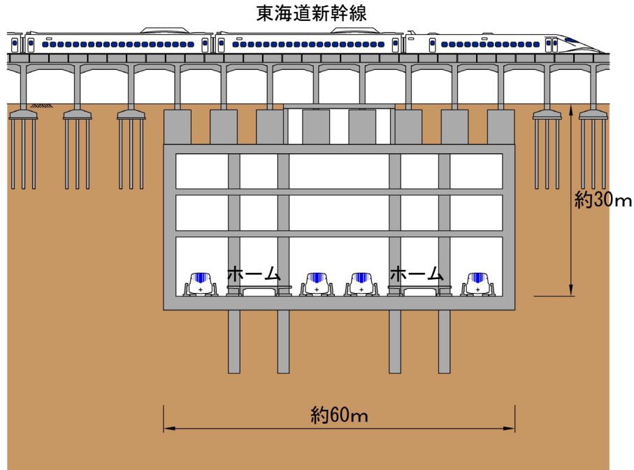
トンネルの標準的な断面図 (都市トンネル)
