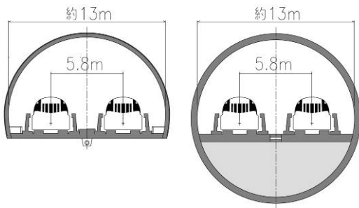
山岳トンネル
