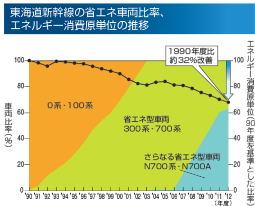
図 19-3-2-1 東海道新幹線の省エネ車両比率、エネルギー消費原単位の推移
