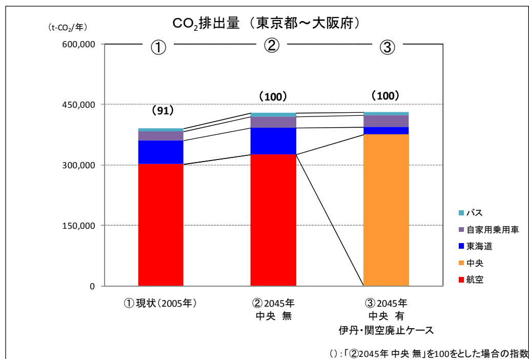
図 19-2-1-5 各ケースにおける CO 2 排出量 (東京都～大阪府間)
