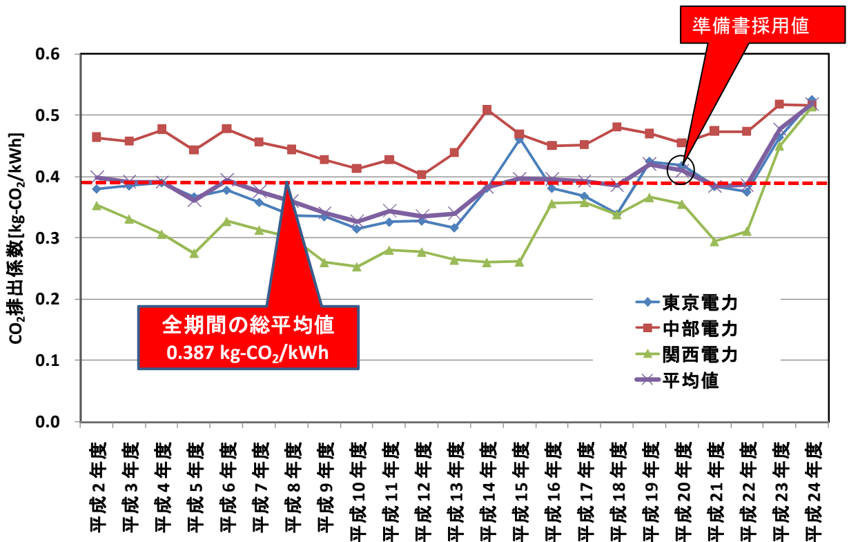
図 19-2-3-1 電力会社のCO 2 排出係数の状況
