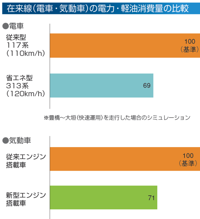
図 19-3-2-4 在来線（電車・気動車）の電力・軽油消費量の比較
