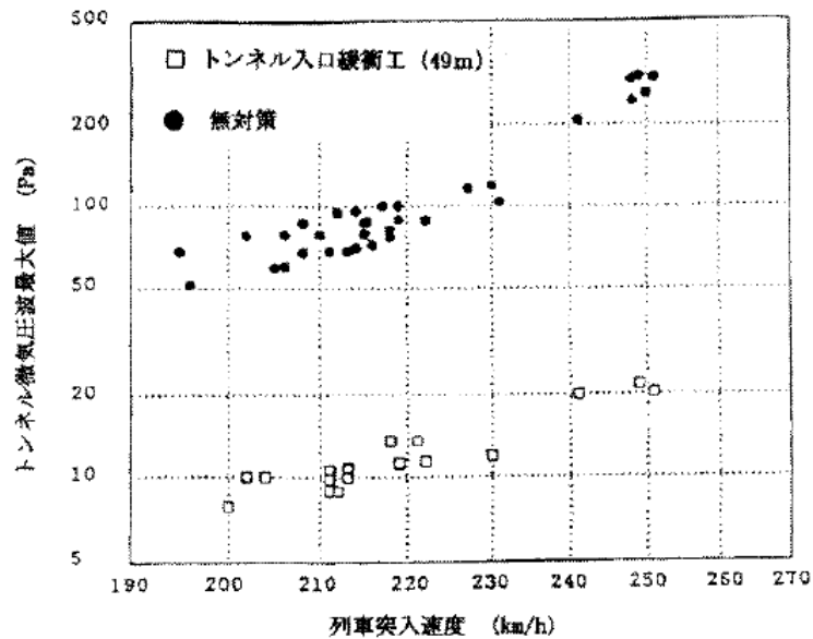
図 4-3-1-1 トンネル緩衝工（長さ 49m）のトンネル微気圧波低減効果
