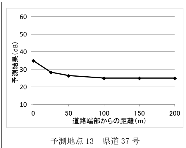
図 3-5-2 (3) 資材及び機械の運搬に用いる車両の運行に係る振動の距離減衰の状況
