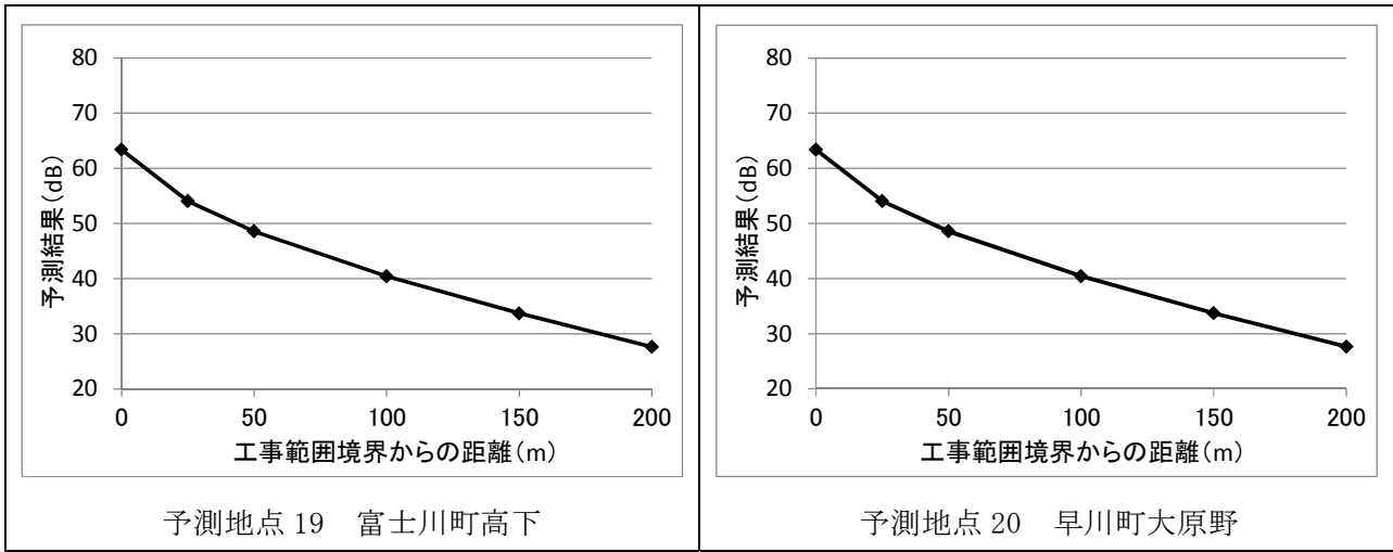
図 3-5-1 (4) 建設機械の稼働に係る振動の距離減衰の状況
