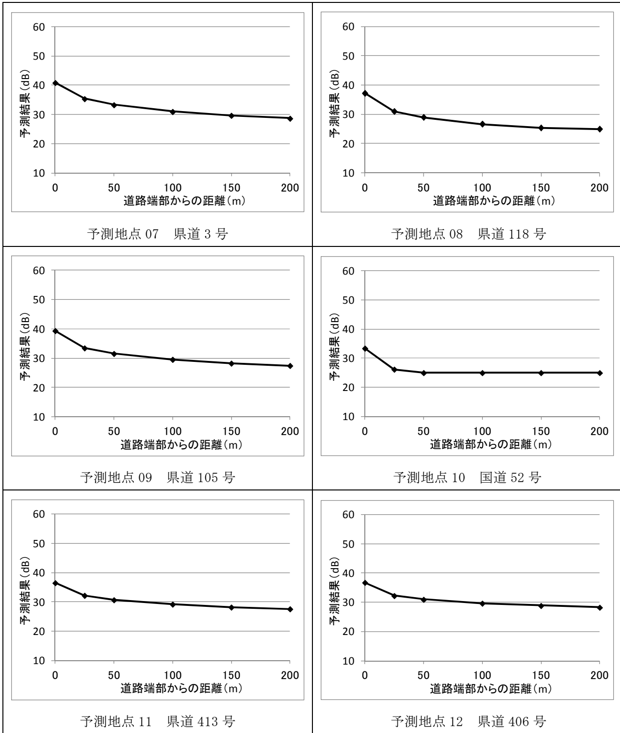
図 3-5-2(2) 資材及び機械の運搬に用いる車両の運行に係る振動の距離減衰の状況
