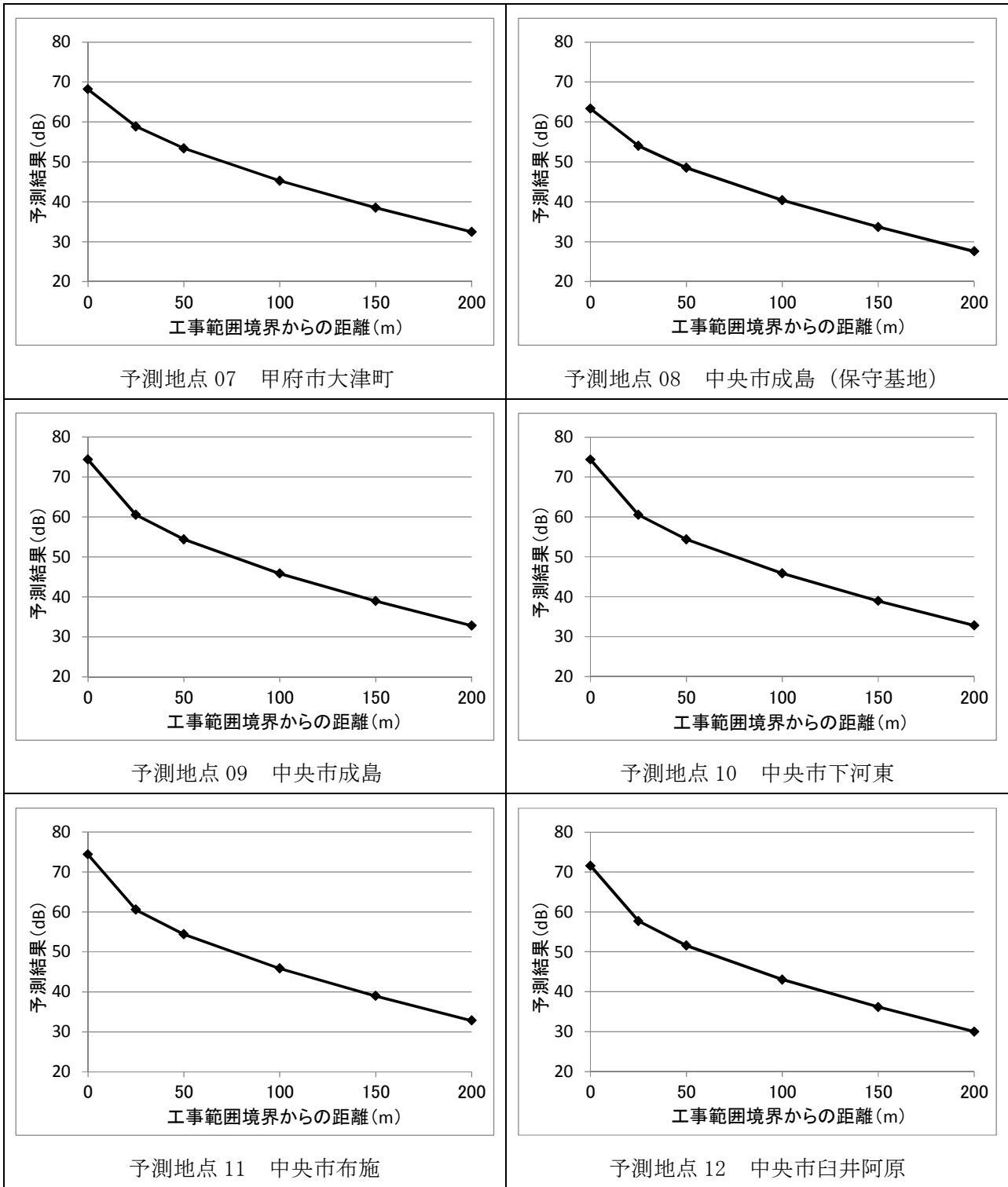
図 3-5-1 (2) 建設機械の稼働に係る振動の距離減衰の状況
