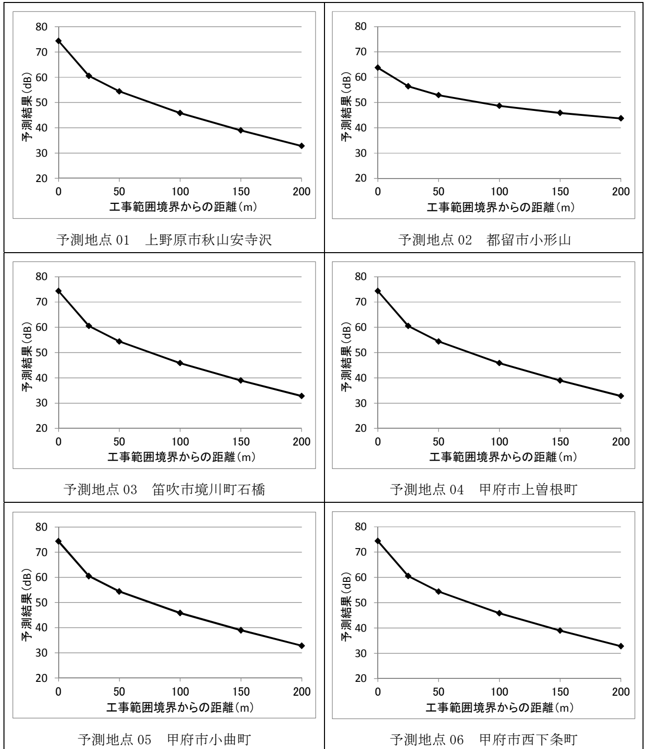
図 3-5-1(1) 建設機械の稼働に係る振動の距離減衰の状況
