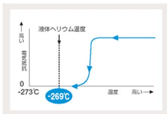
図 3-4-20 電気抵抗と温度の関係
