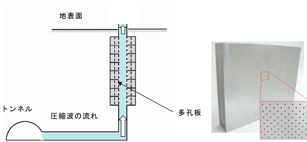
図 4-3-2-1 多孔板の構造
