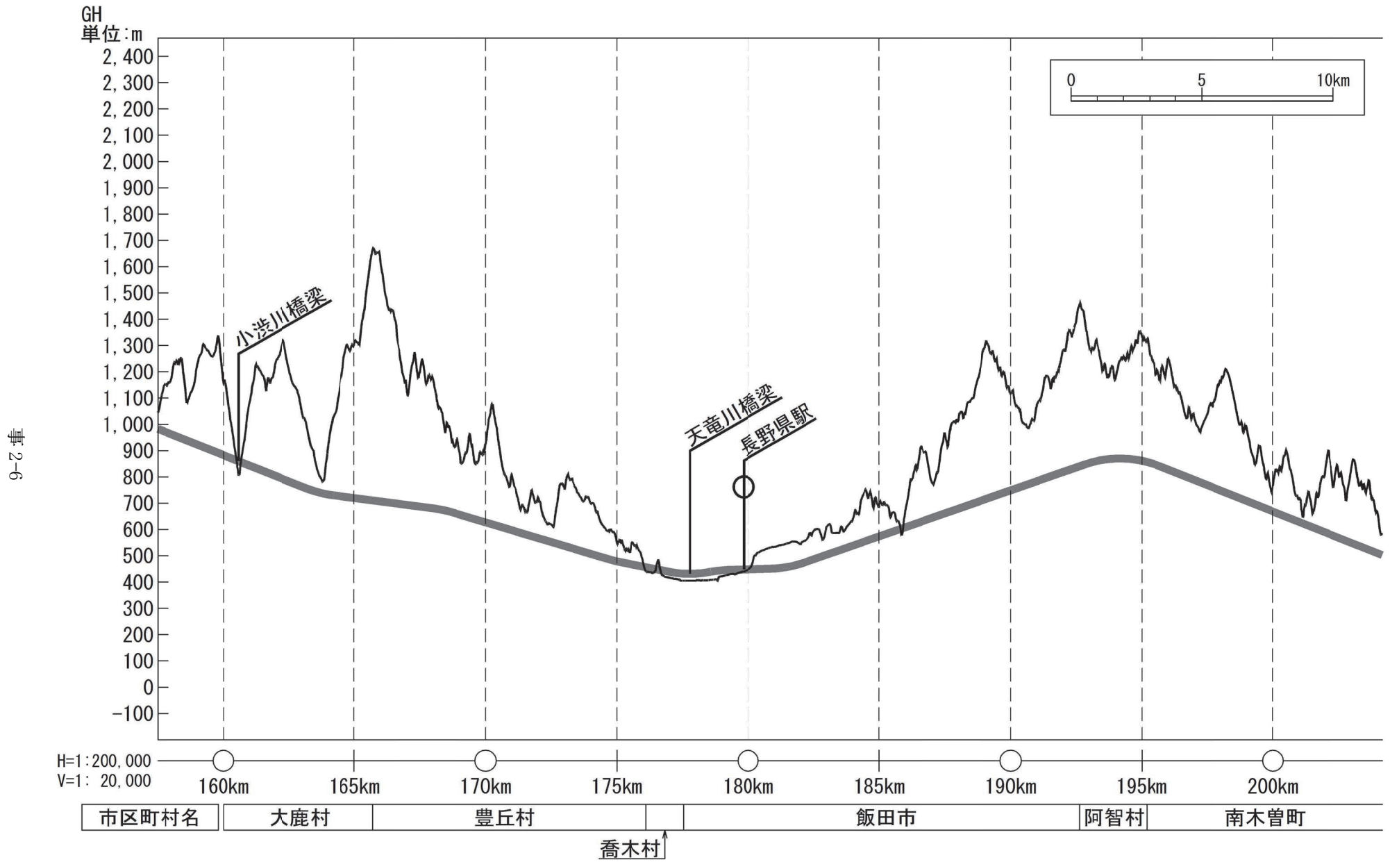
図 2-1 (5) 路線概要 (縦断計画)
