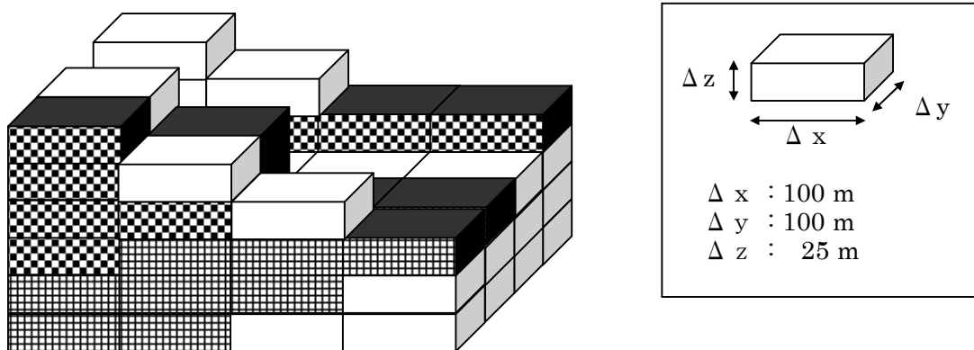
図 8-1-2 モデルの構造のイメージ（直方体ブロックの集合体） （各ブロックの模様の違いで地質の違いを表現している）
