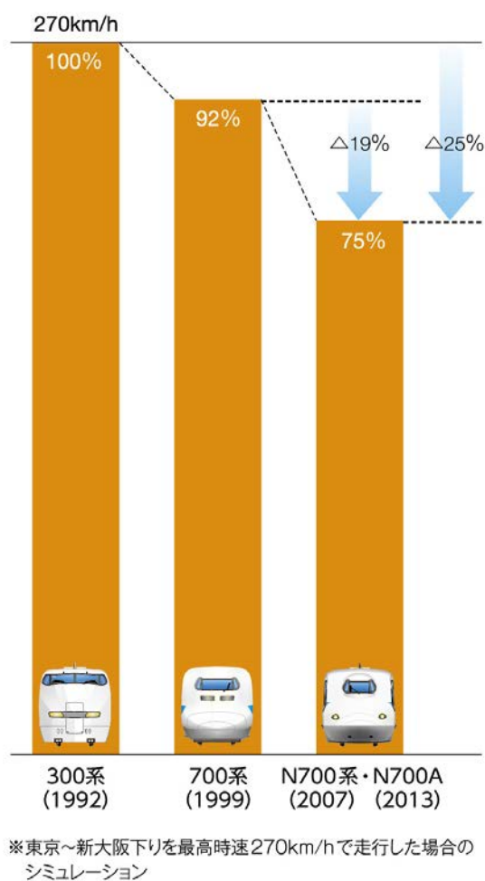
図 19-3-2-3 東海道新幹線の車種別電力消費量の比較
