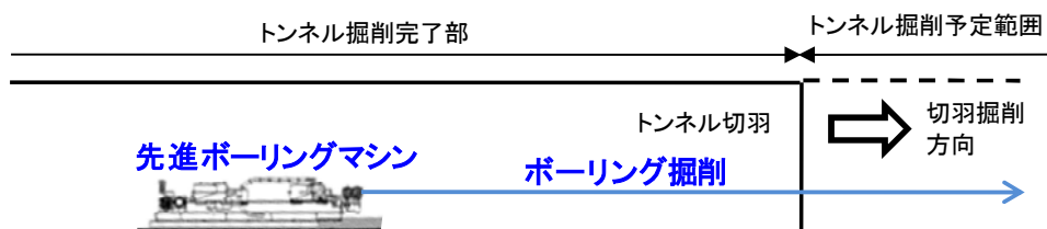
図 7-4-1 先進ボーリングマシンの施工イメージ（断面図）
