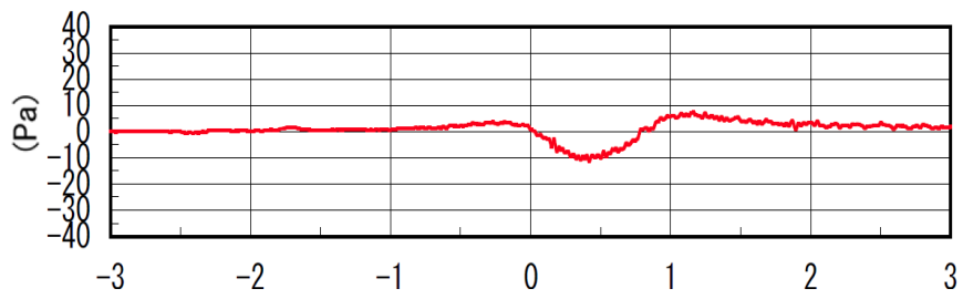
図 5-1-1(2) 防音壁区間での圧力変動の測定値 (50m 離れ)
