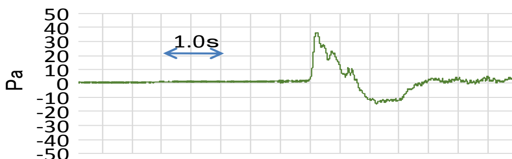
図 4-4-1 微気圧波測定値（20m 離れ）
