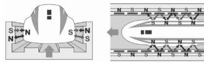
図-1 超高速鉄道の推進・浮上の原理
