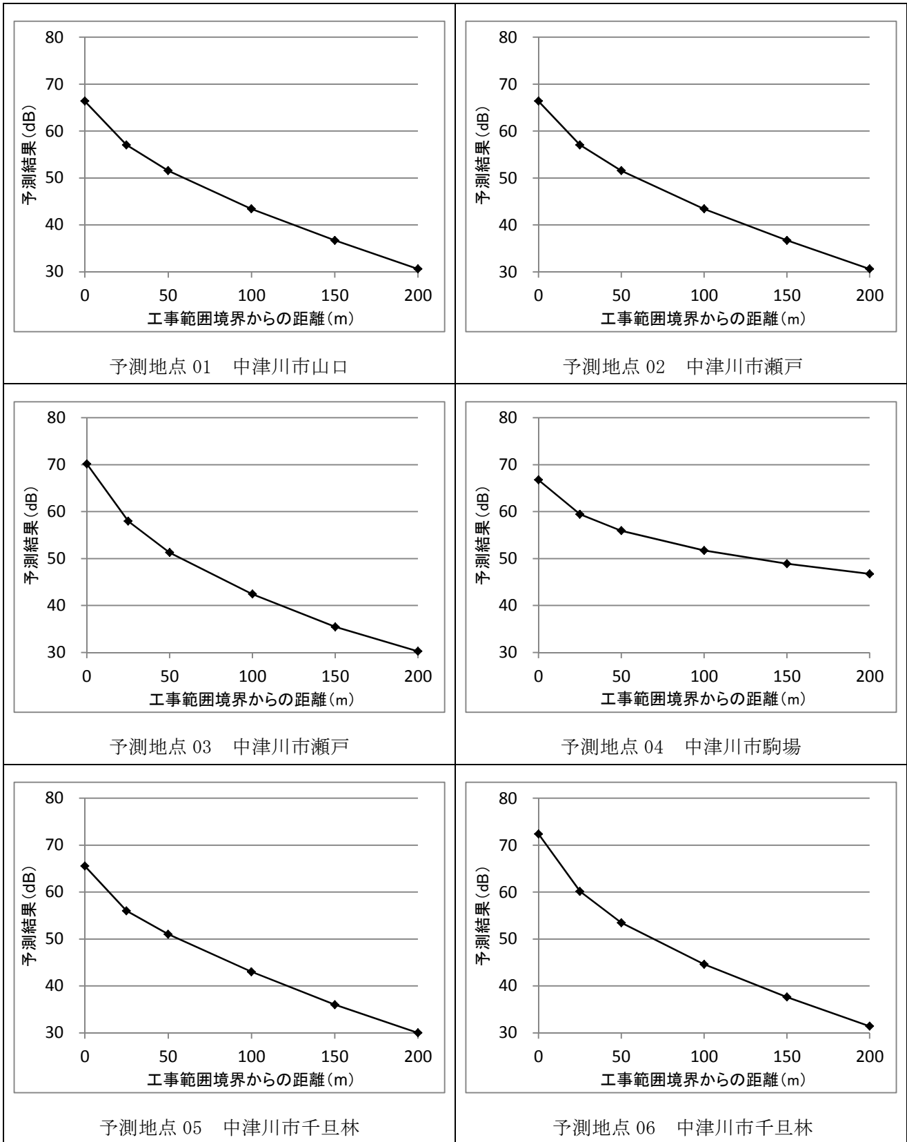
図 3-5-1 (1) 建設機械の稼働に係る振動の距離減衰の状況
