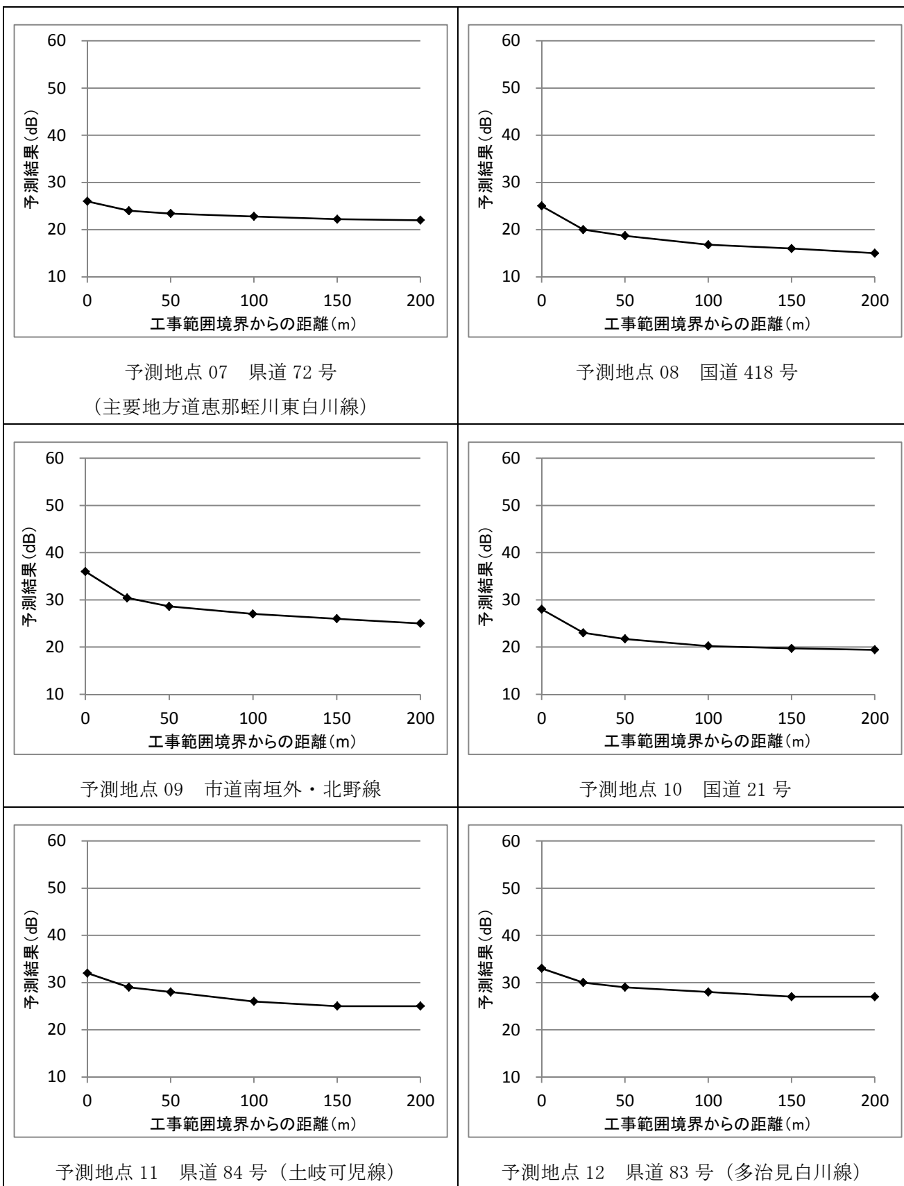
図 3-5-2(2) 資材及び機械の運搬に用いる車両の運行に係る振動の距離減衰の状況
