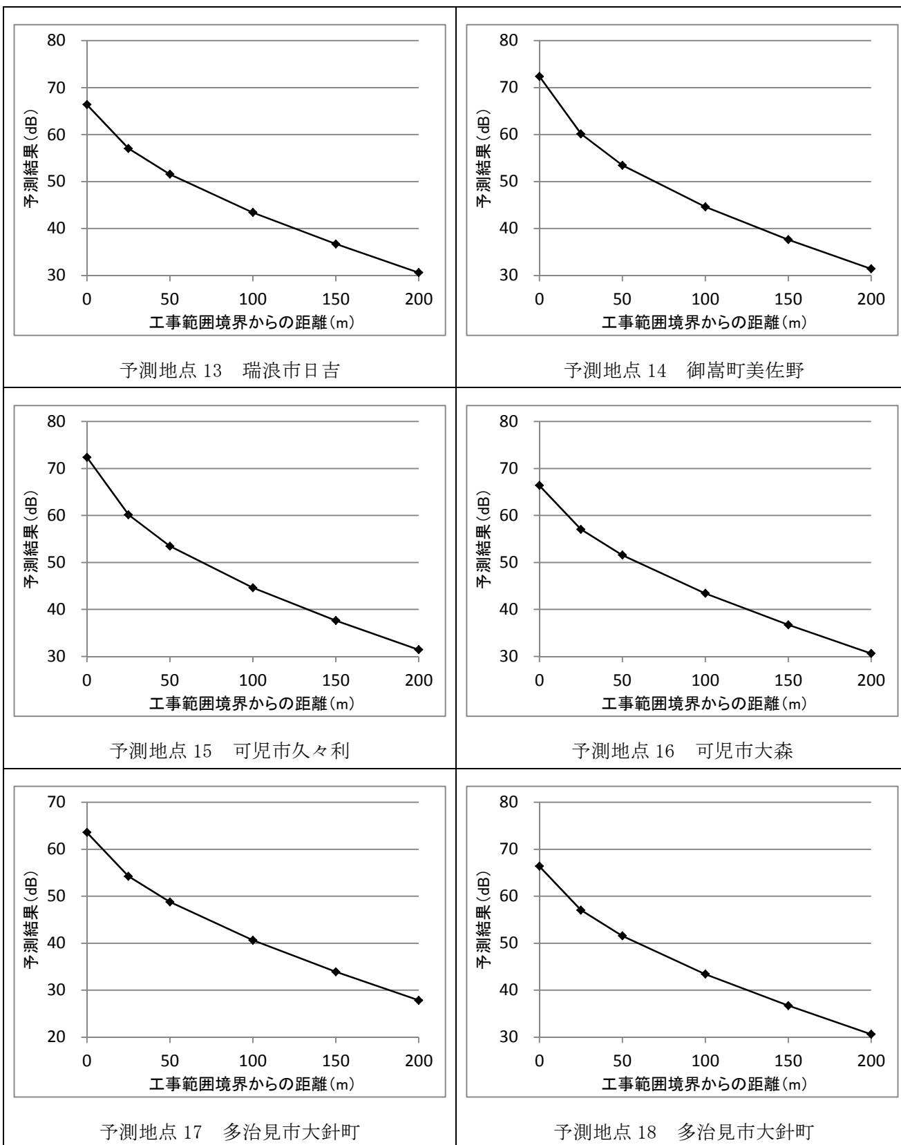
図 3-5-1 (3) 建設機械の稼働に係る振動の距離減衰の状況
