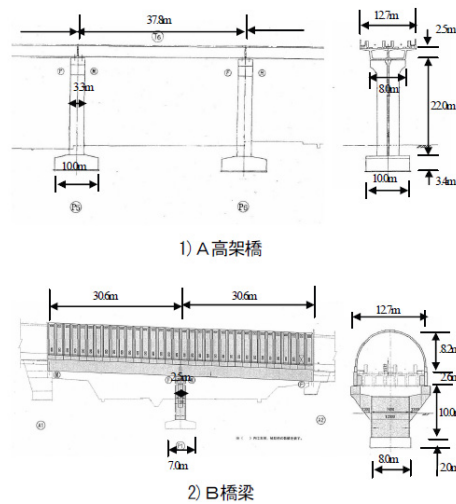
図-2 測定対象構造物の概要
