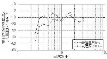
b) 1/3オクターブバンド振動レベル
