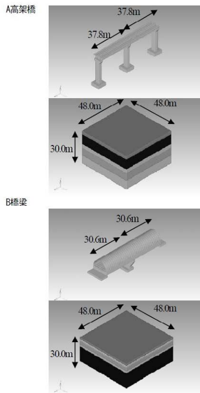
図-23 高架橋及び地盤のボクセルモデル
