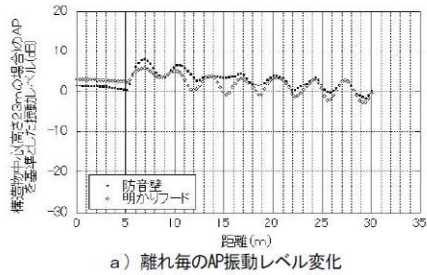
a) 離れ毎のAP振動レベル変化
