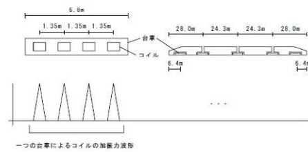
図-24 列車荷重のモデル化概要
