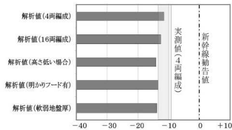
図-33 各ケースの予測結果と新幹線勧告値の比較
