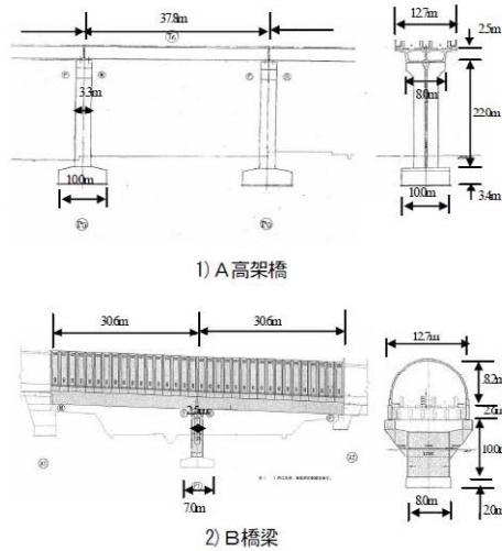
図-2 測定対象構造物の概要
