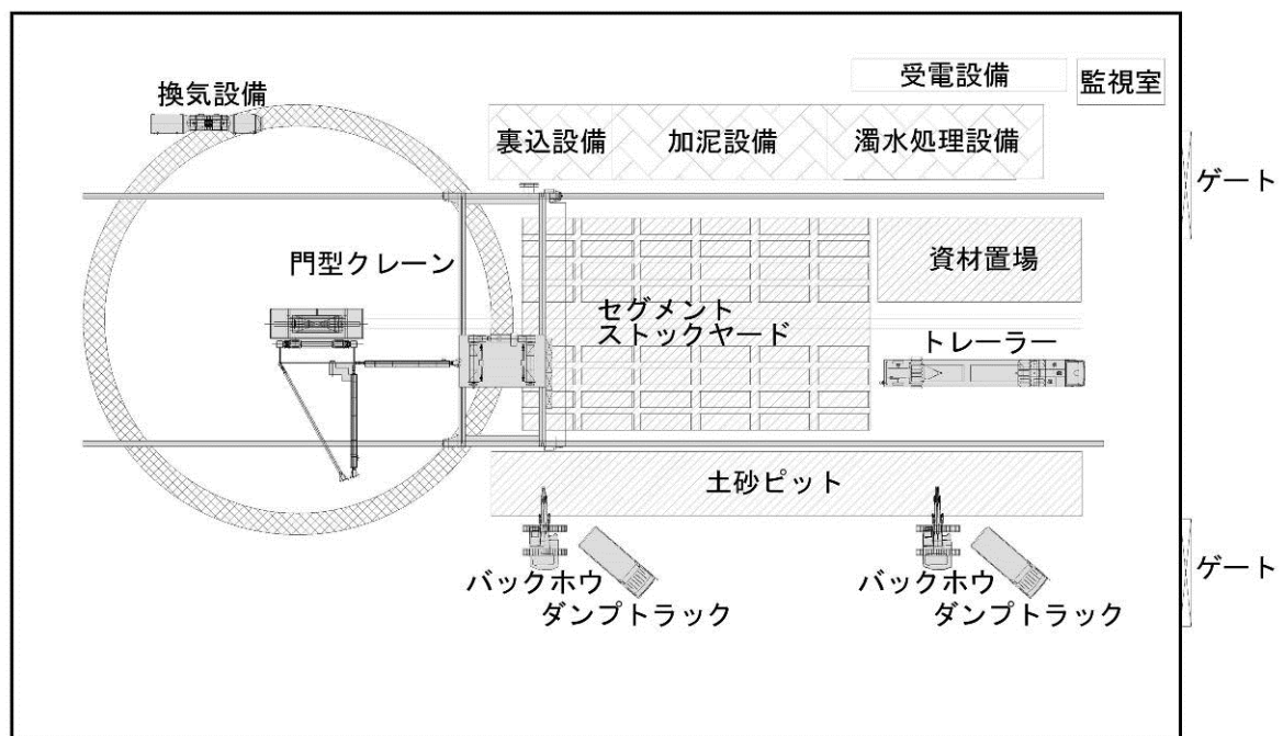
図 3-4-6-22 非常口の施エヤードの概要（土圧式シールド工法によるトンネル施工時）
