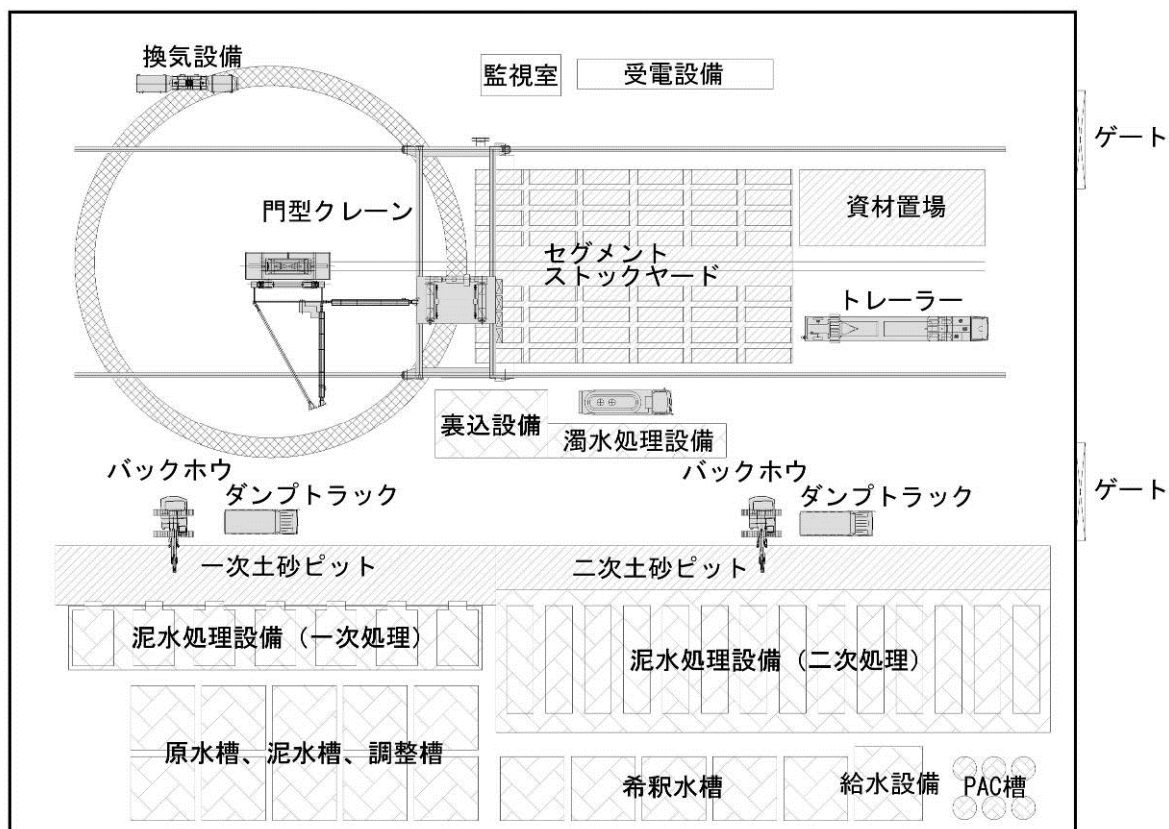
図 3-4-6-21 非常口の施エヤードの概要（泥水式シールド工法によるトンネル施工時）
